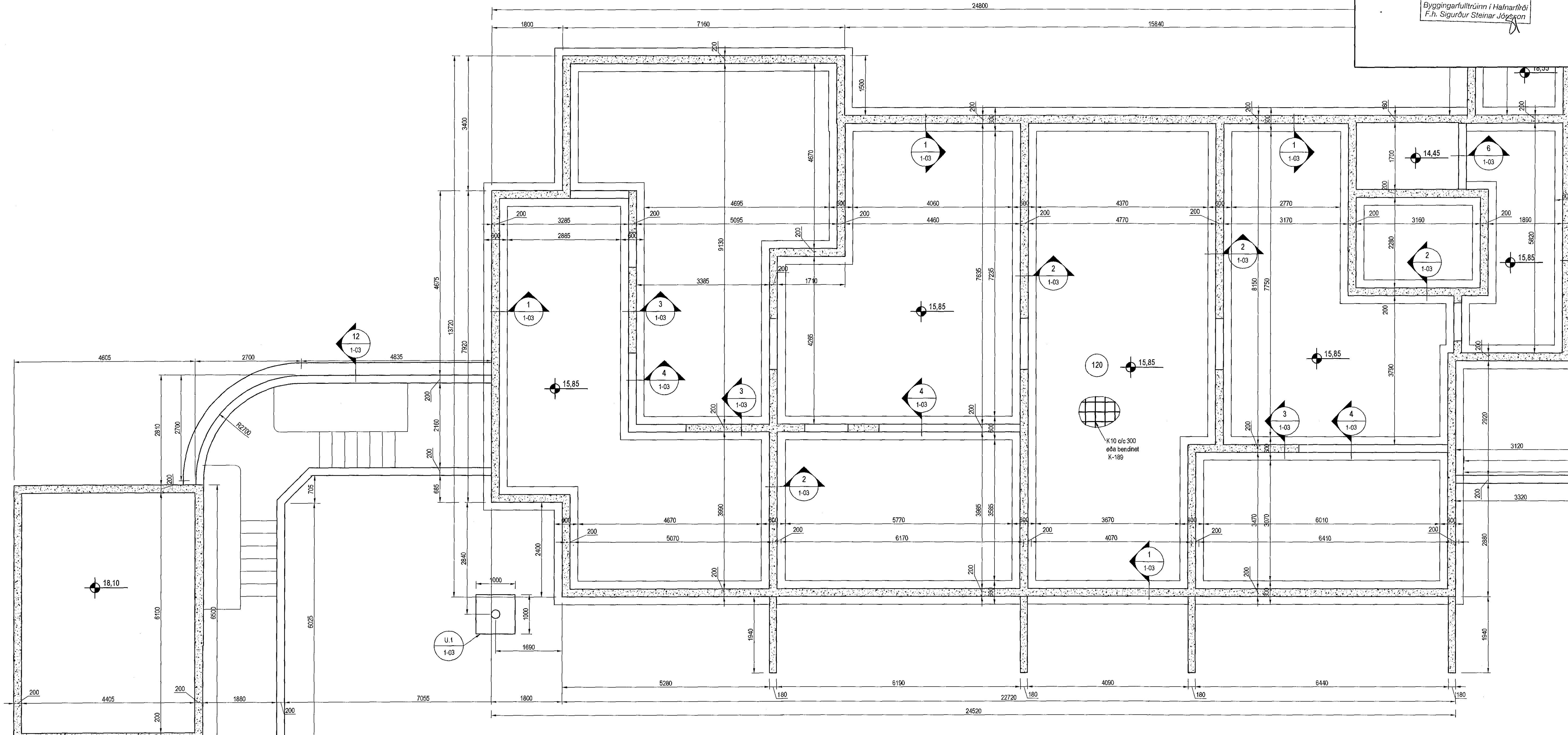
Undirstöður, Grunnmynd, 1:50
