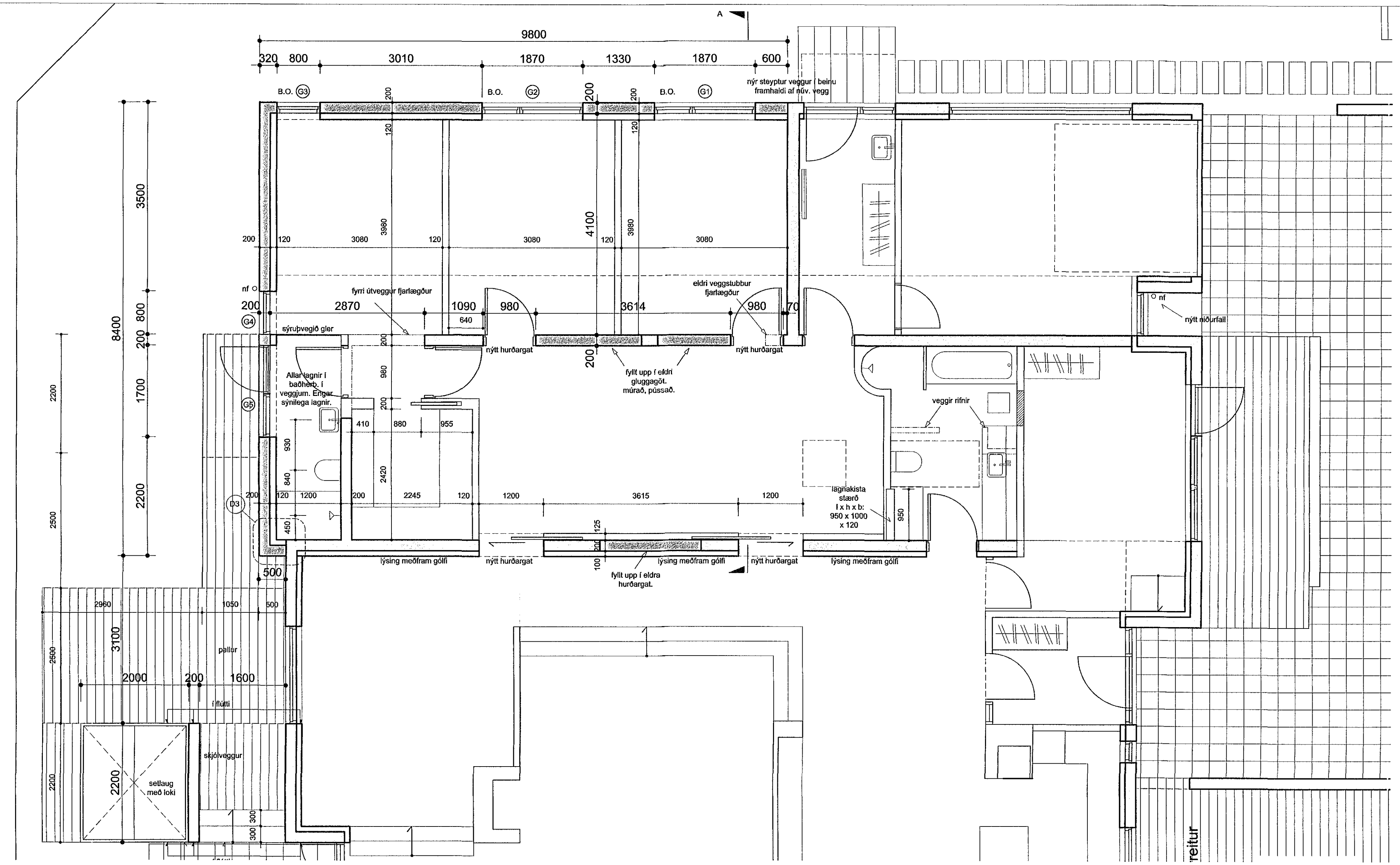
Grunnmynd mkv. 1:50
