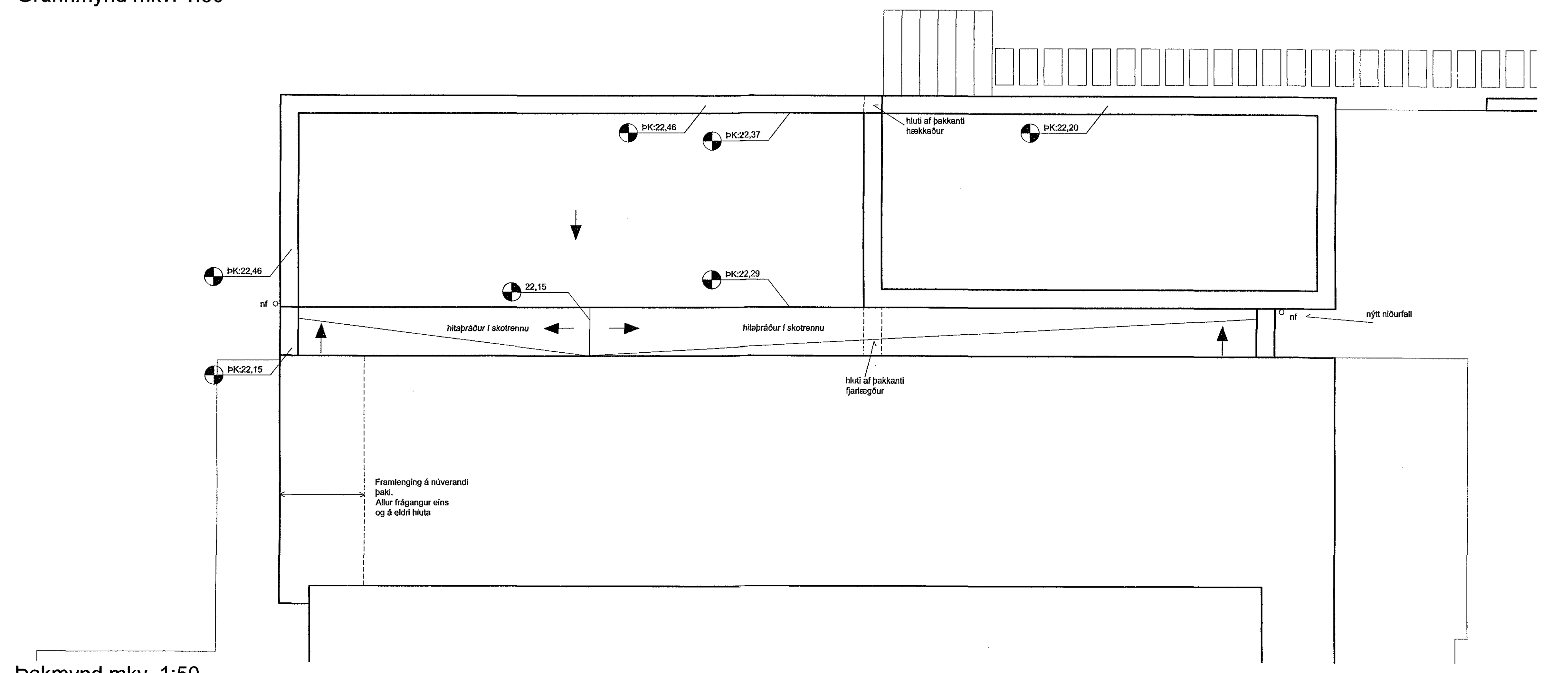
Þakmynd mkv. 1:50
