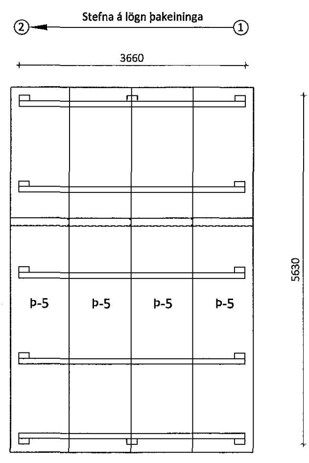
Þakmynd Mkv. 1:60
