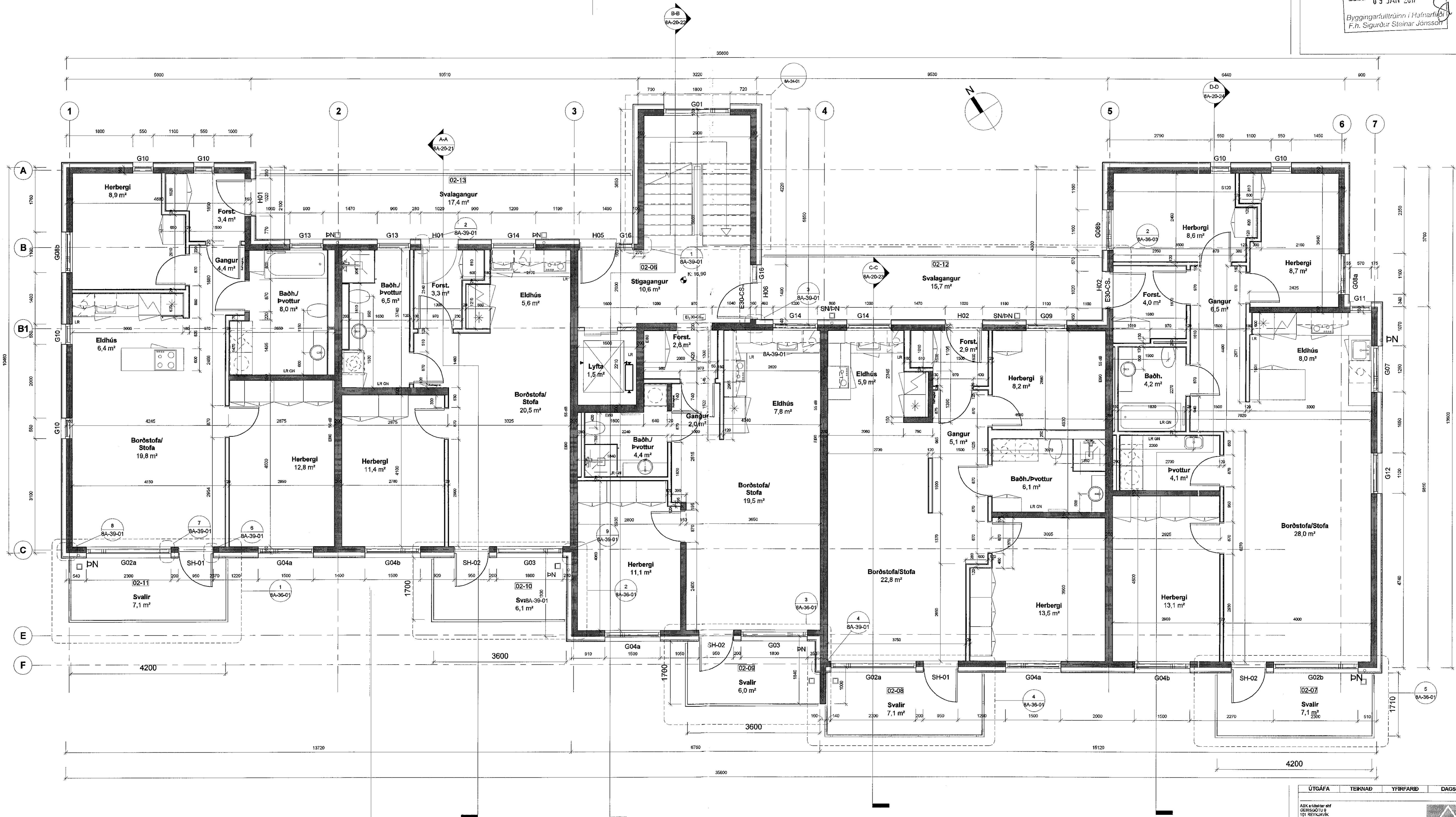
1 Hæð 2 50 - 8A 1 : 50
