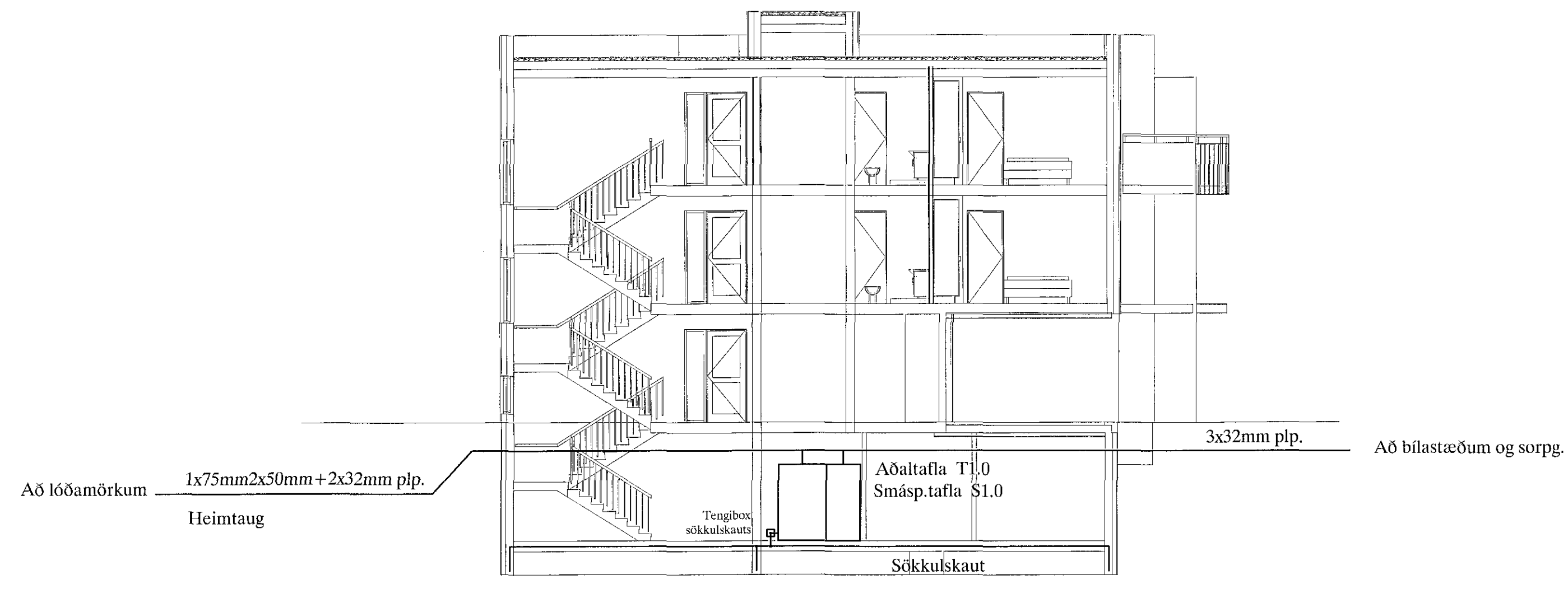
SNÍÐ Í INNTAK M. 1:100
