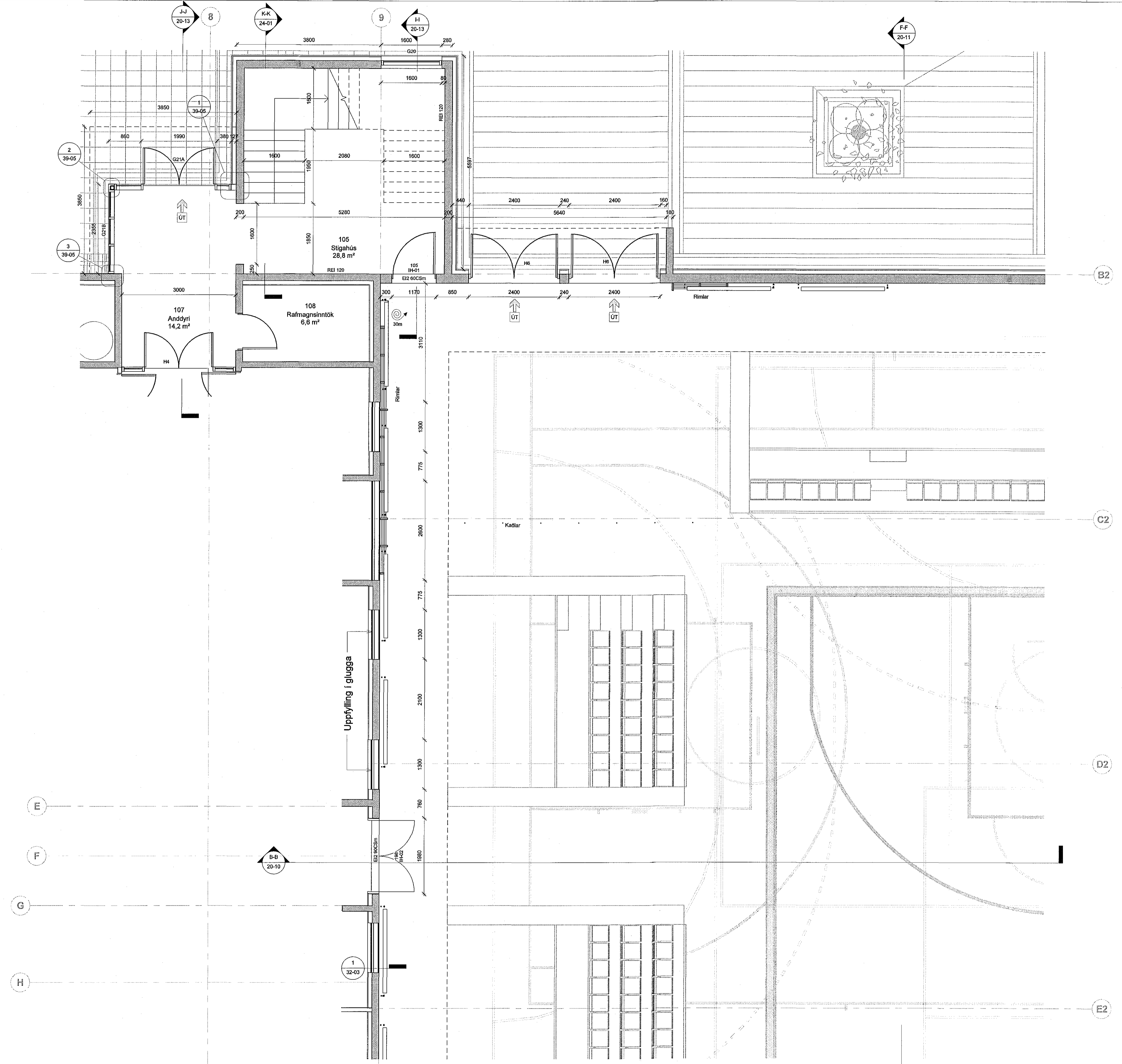
1. hæð - grmd 50 - hluti 1 1 : 50
