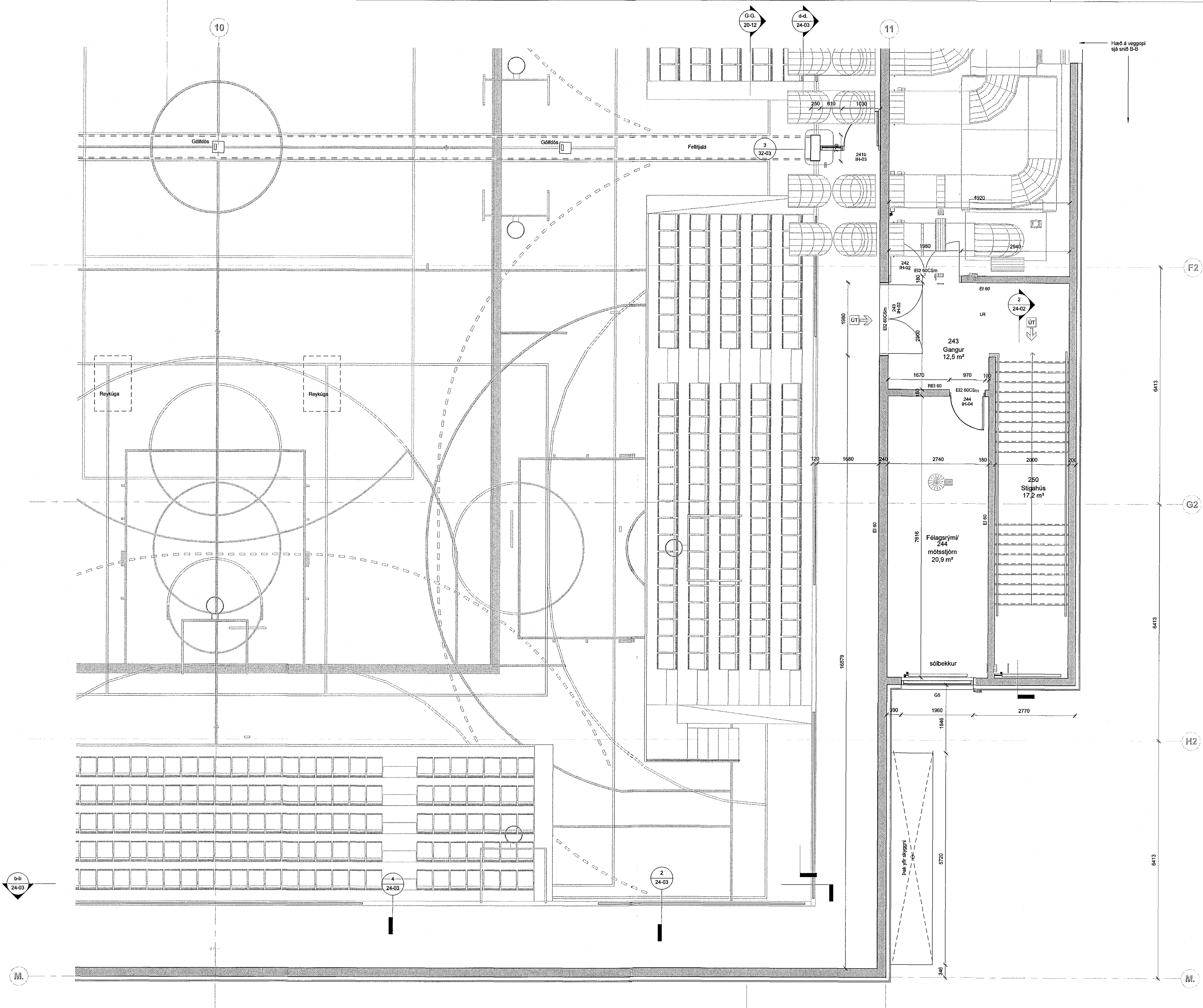
2.hæð - grnd 50 - hluti 4 1:50
