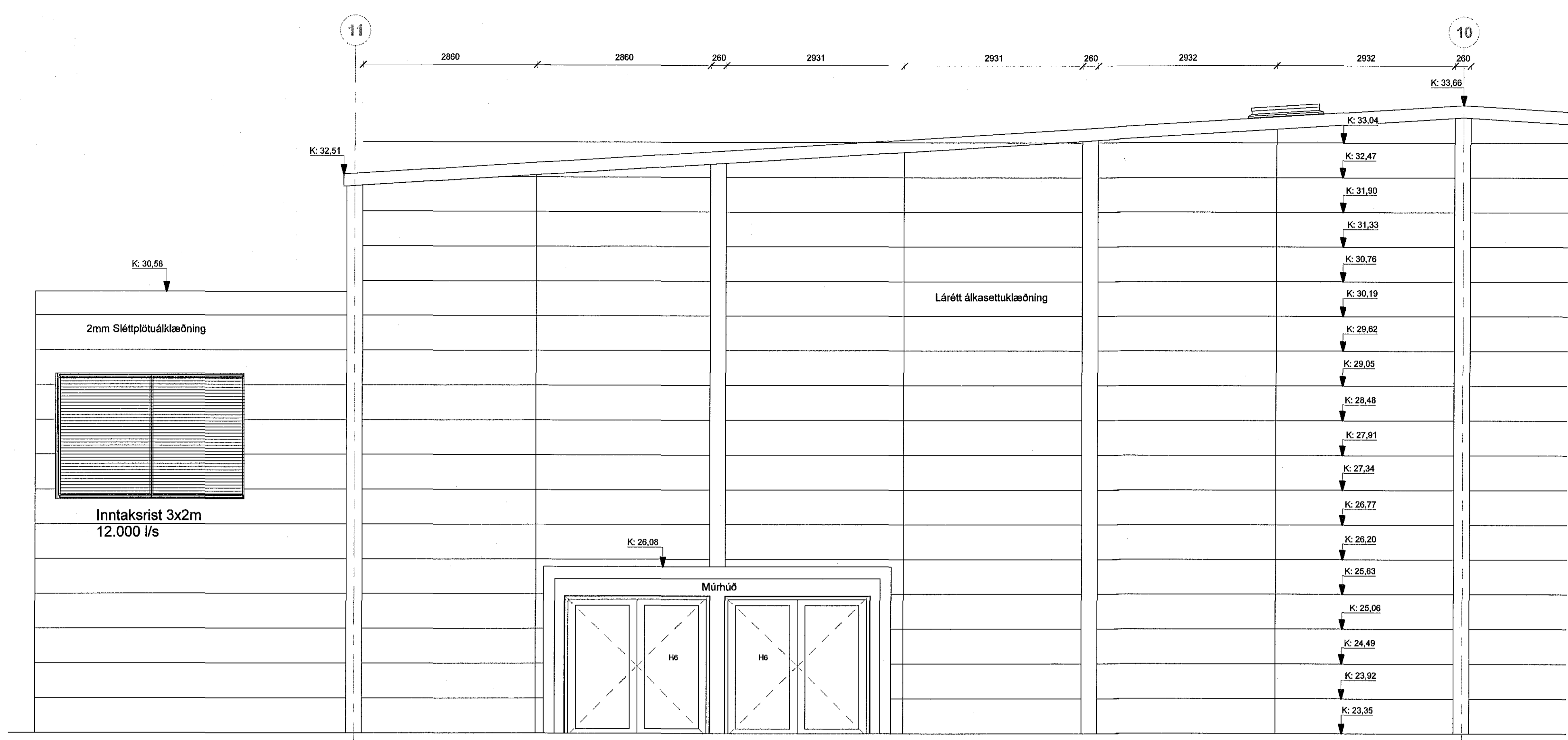
Norður 50 - hluti 1 1 : 50
