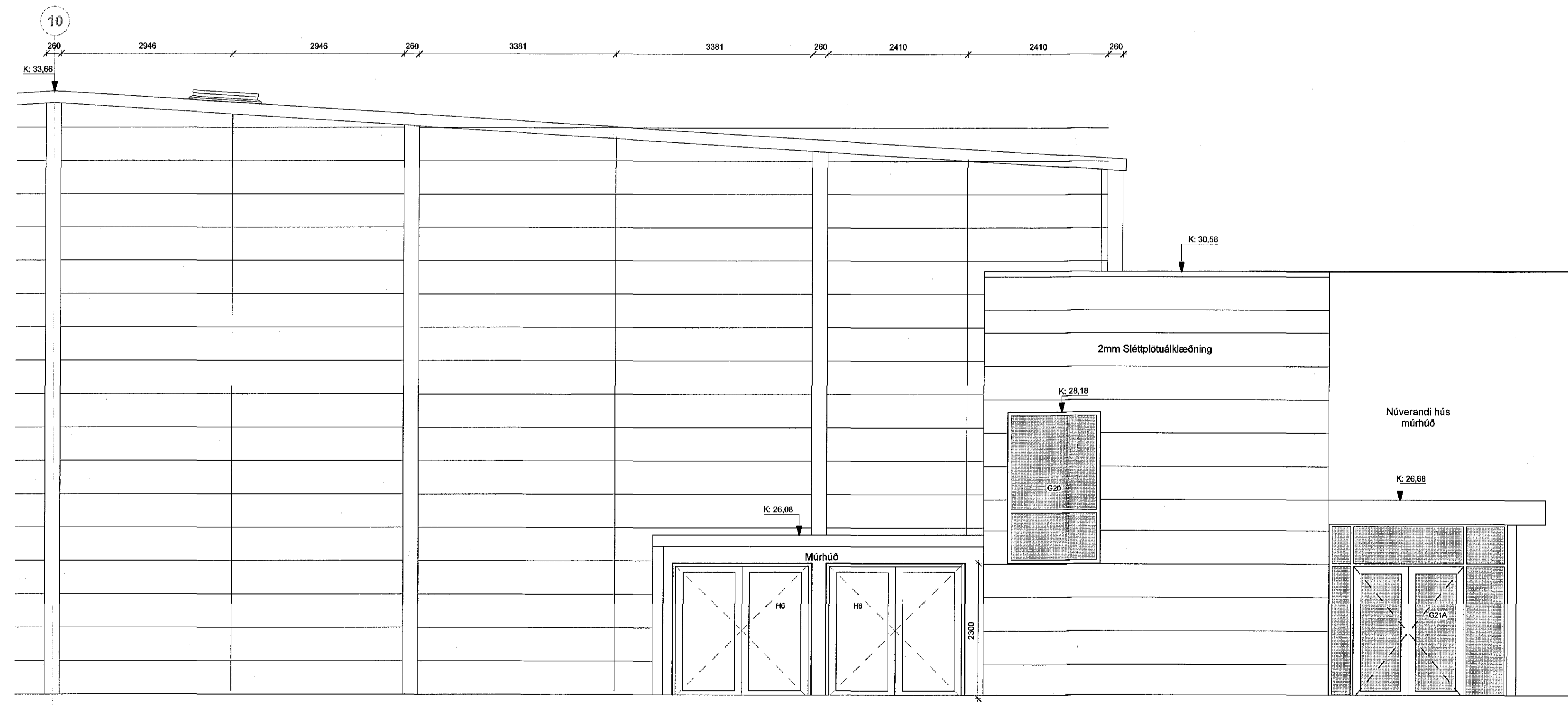
Norður 50 - hluti 2 1 : 50
