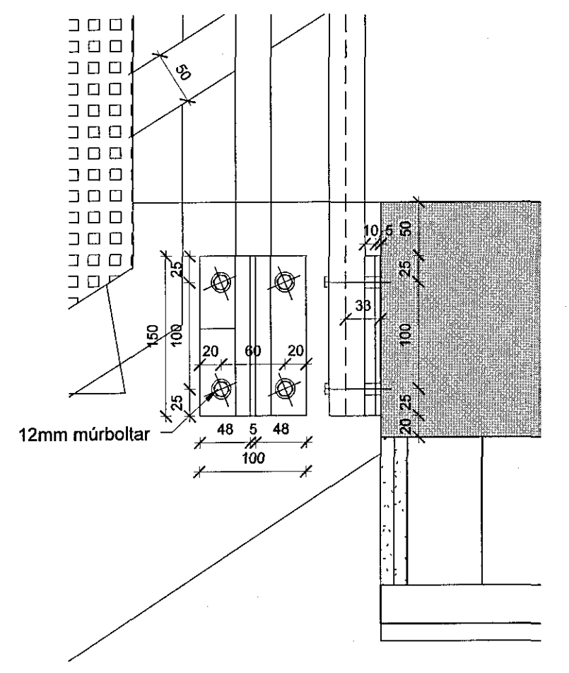
Grunnmynd stigi norður 1:20
