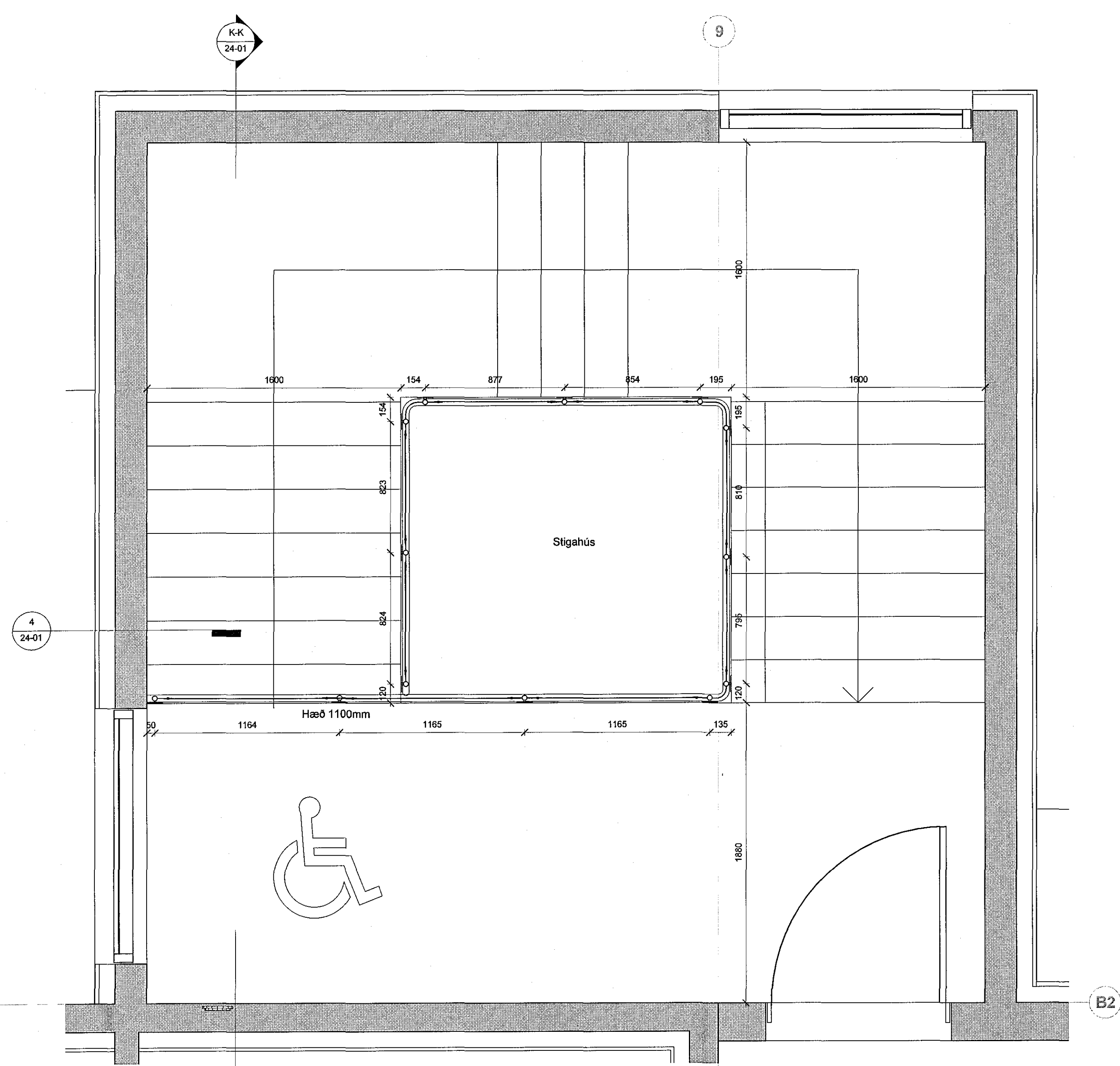
Grunnmynd stigi norður 1:20
