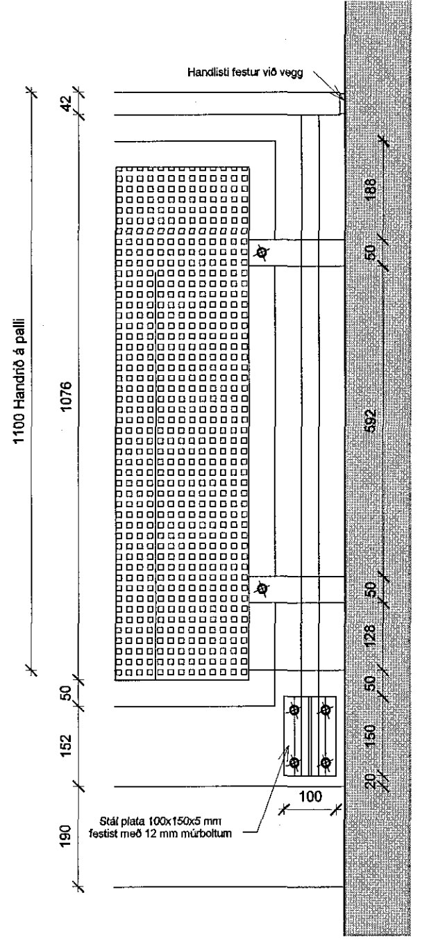
Stigahandrið ásýnd 1:10
