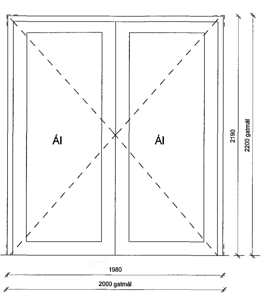
Flóttaleið, paníkslá
