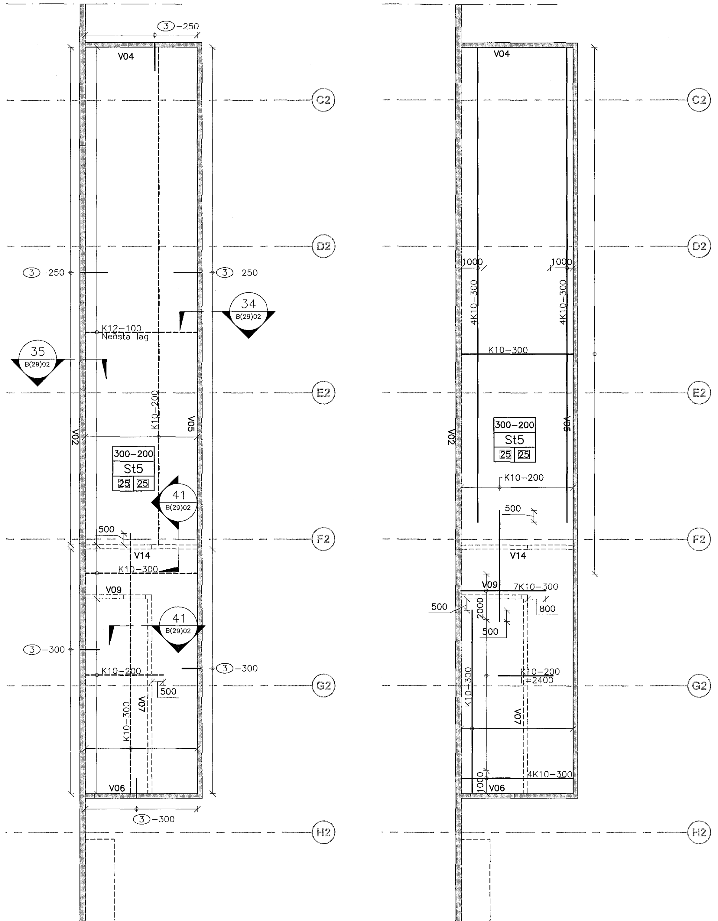
Járnbanding í neðri brún þaks yfir tæknirými Mkv: 1:100
