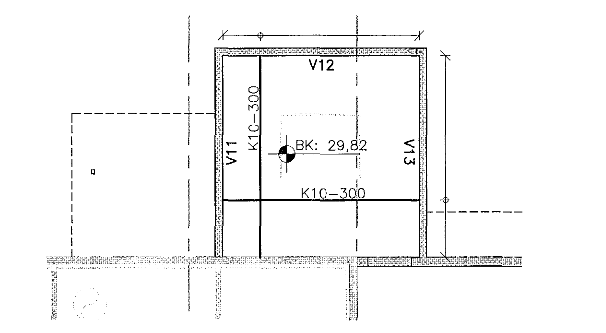
Járnbanding efri brún í þakplötu stigahúss Mkv: 1:100
