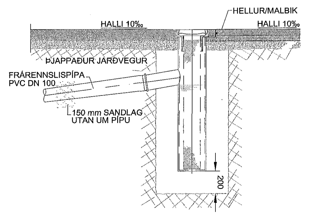
DÆMIGERÐUR FRÁGANGUR Á NIDURFALLI 1:20
