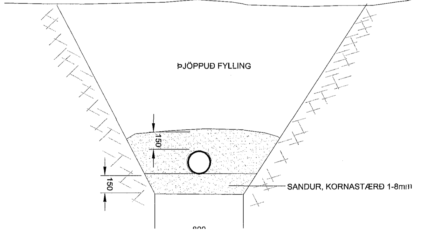
DÆMIGERT SNIÐ Í LAGNASKURD 1:20
