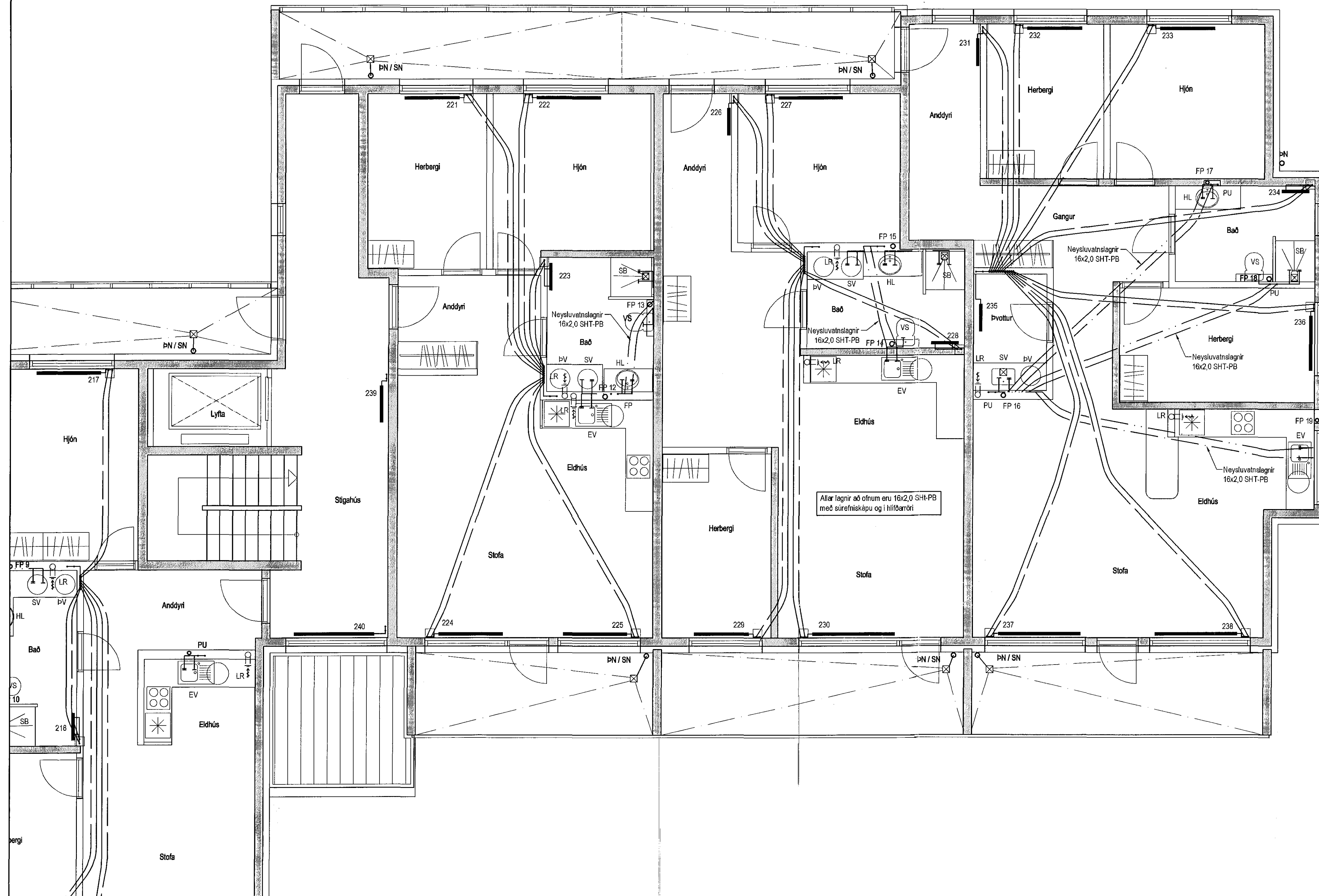
Lagnir 2. hæð, Grunnmynd 1:50
