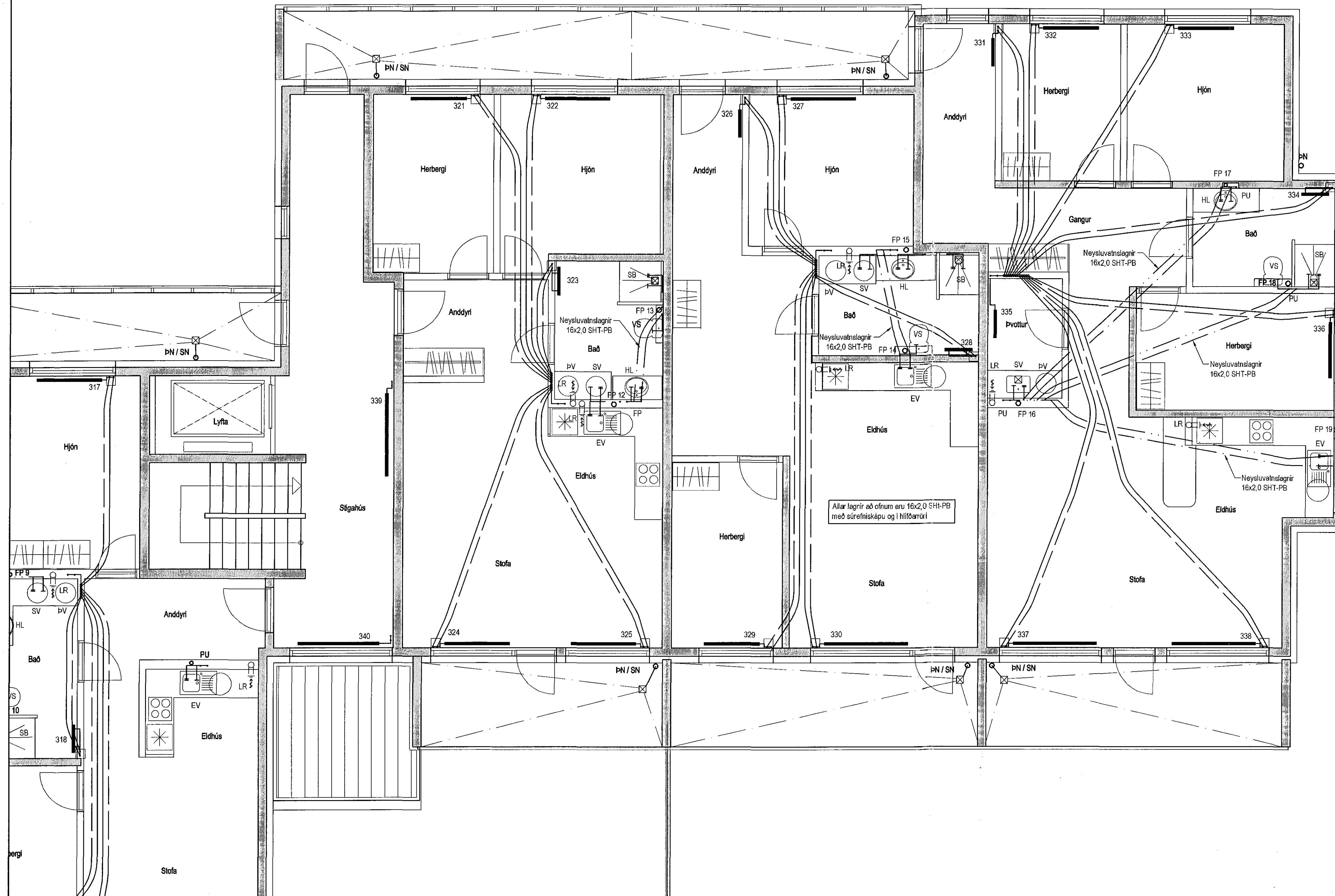
Lagnir 3. hæð, Grunnmynd 1:50
