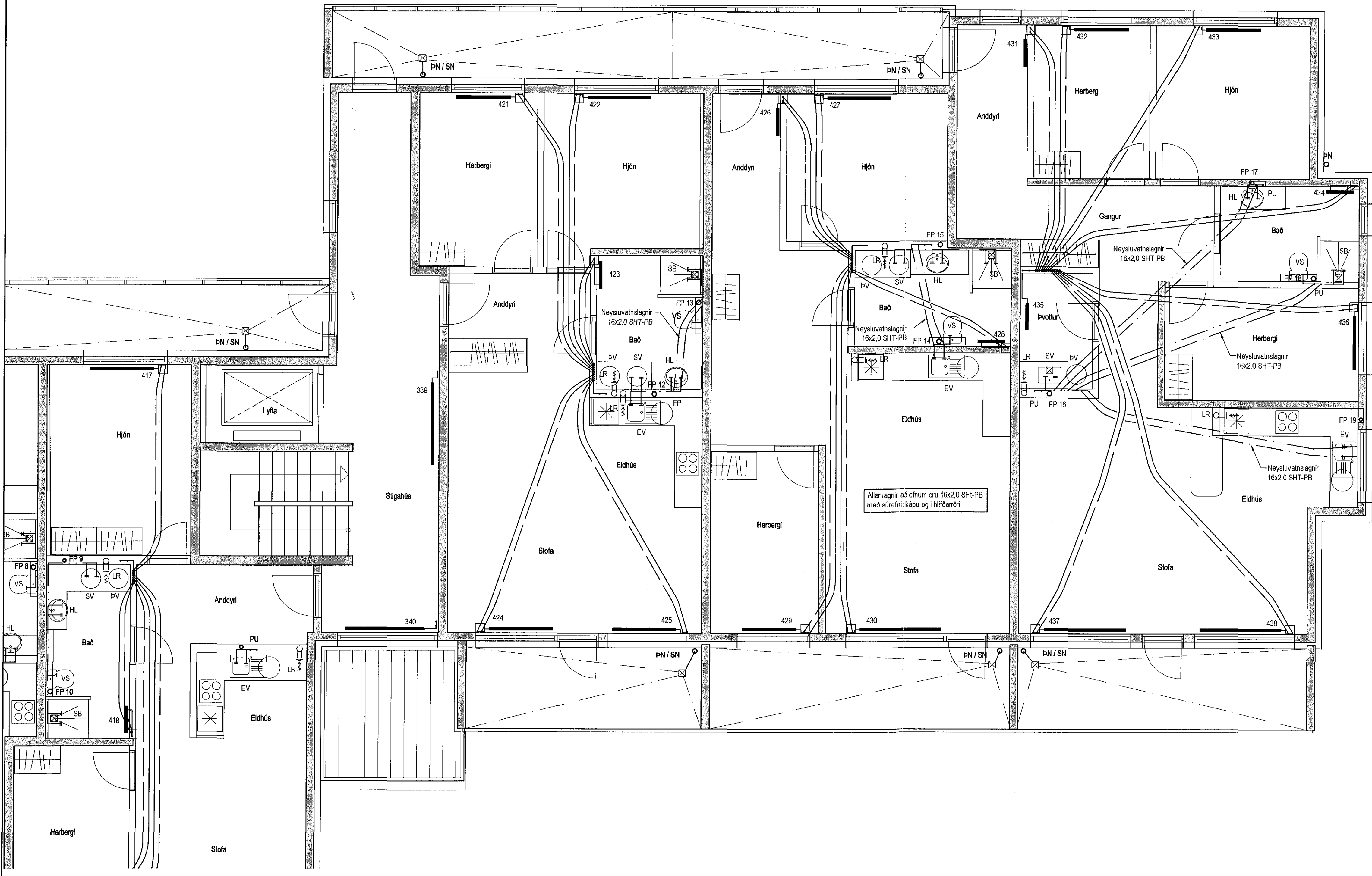
Lagnir 4. hæð, Grunnmynd 1:50
