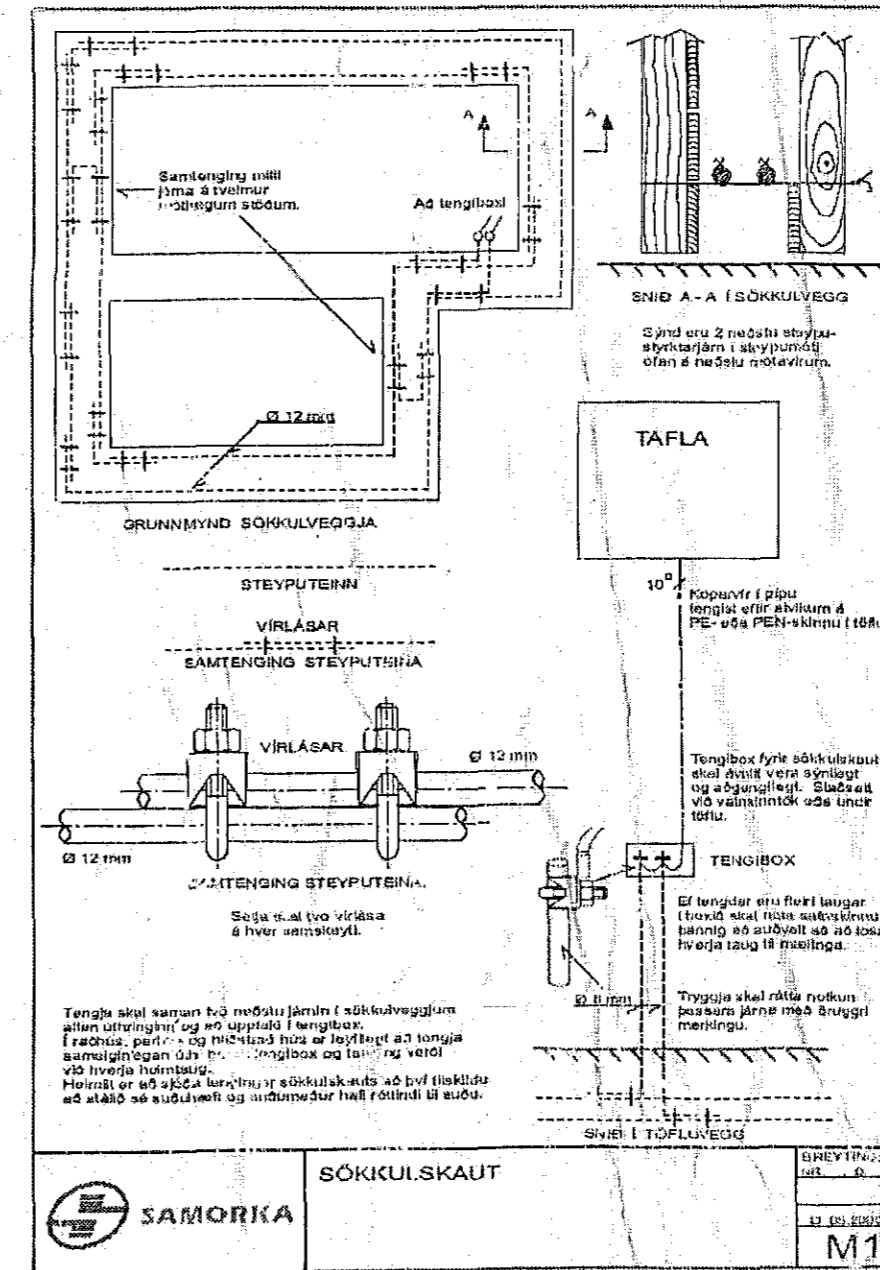
FRÁGANGUR SÖKKULSKAUTS
