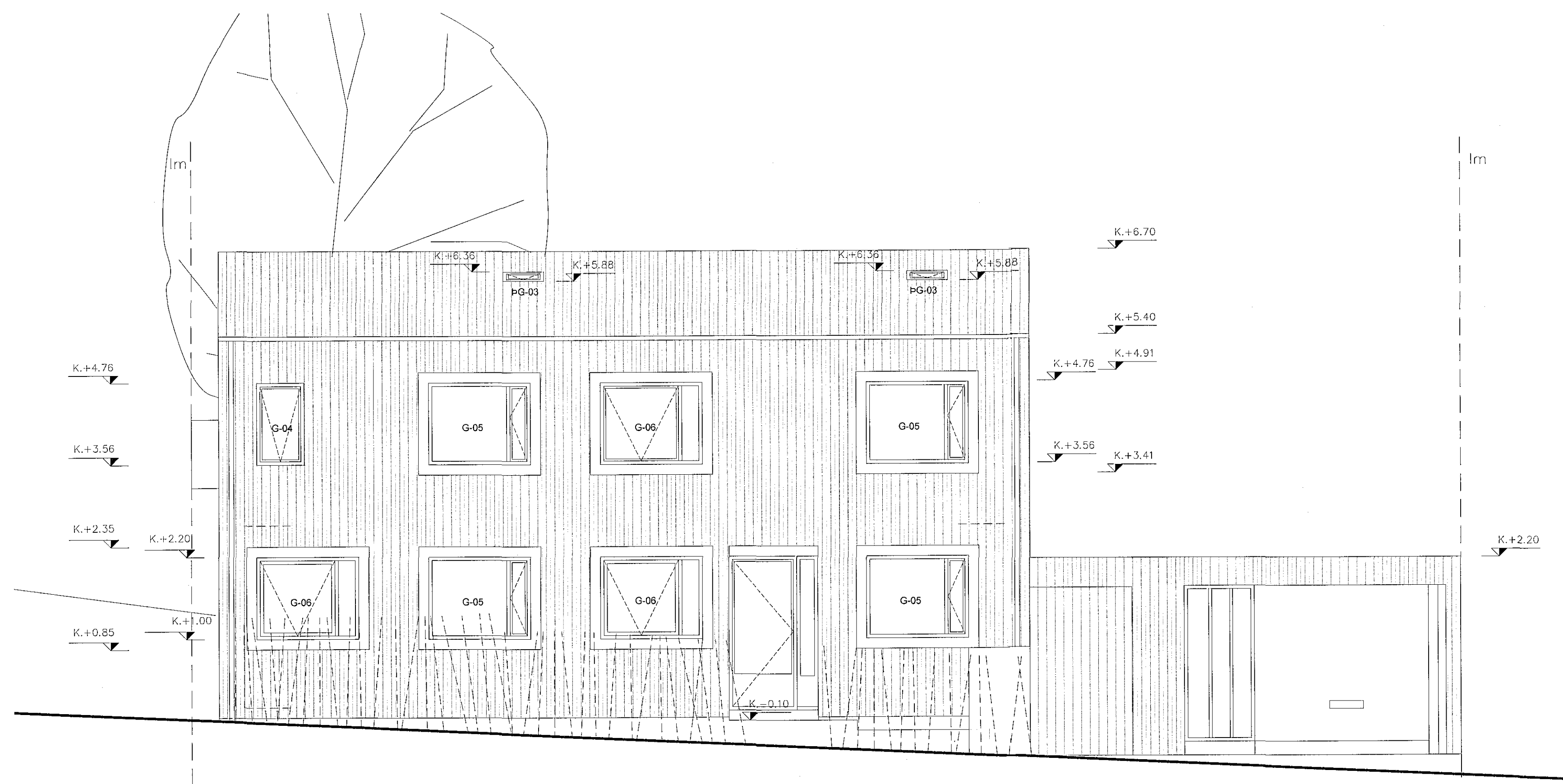
ÚTLIT VESTUR
