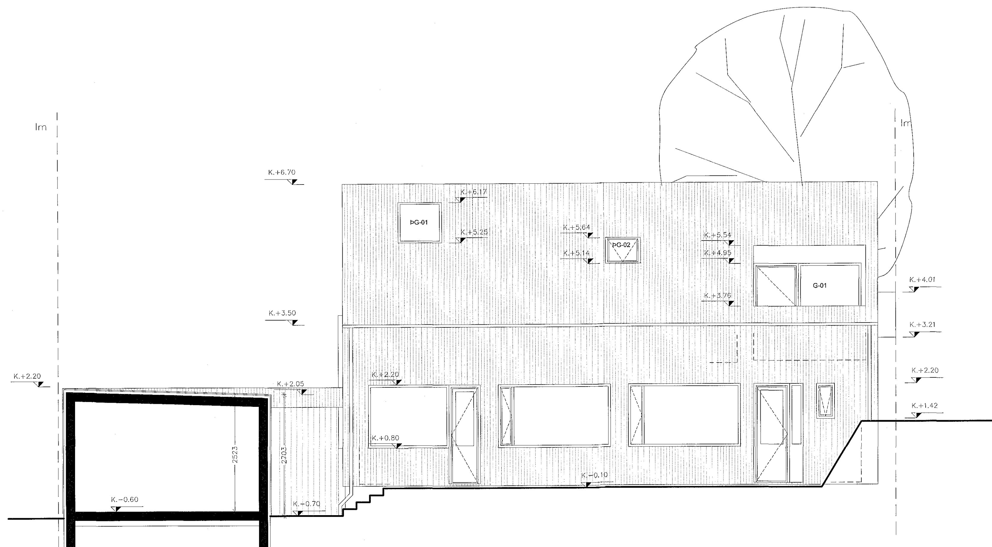
ÚTLIT VESTUR
