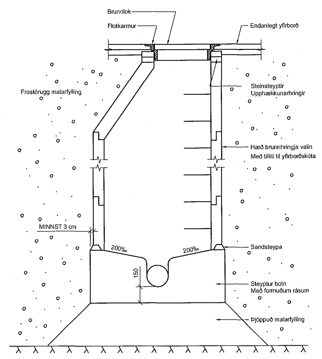
SM1 Skolpbrunnur, 1:20 Dæmigert þversnið
