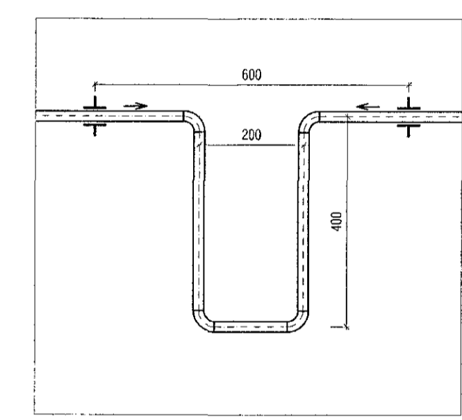
SNIÐ Í ÞENSLUHLÝKK
