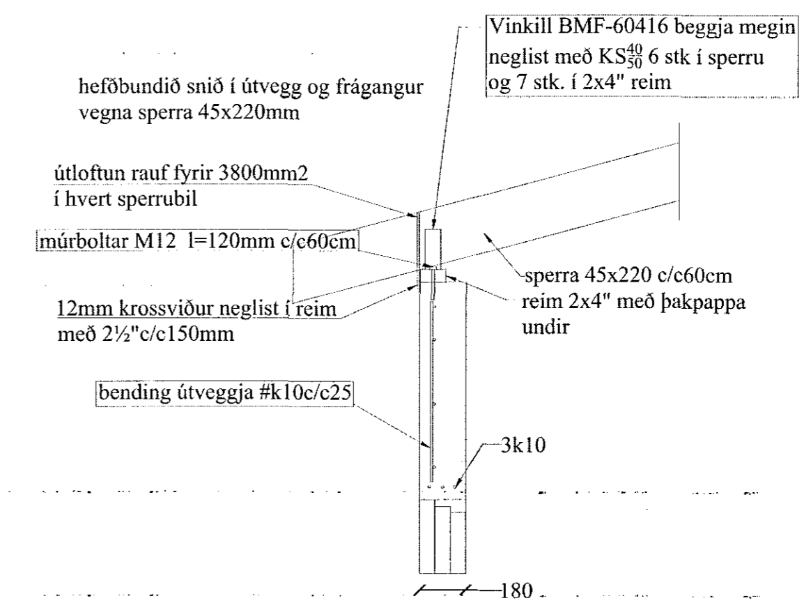
snið B4-B4 mkv. 1:20
