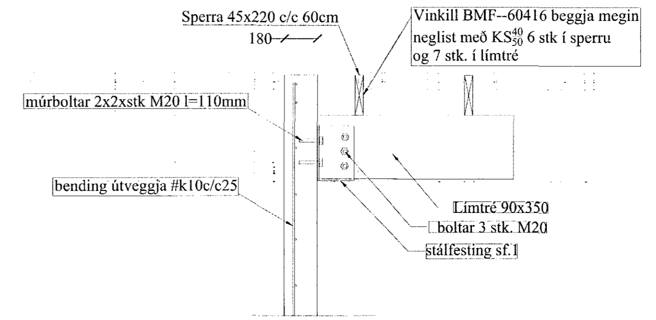
snið B3-B3 stálfasting sf.2 1:20
