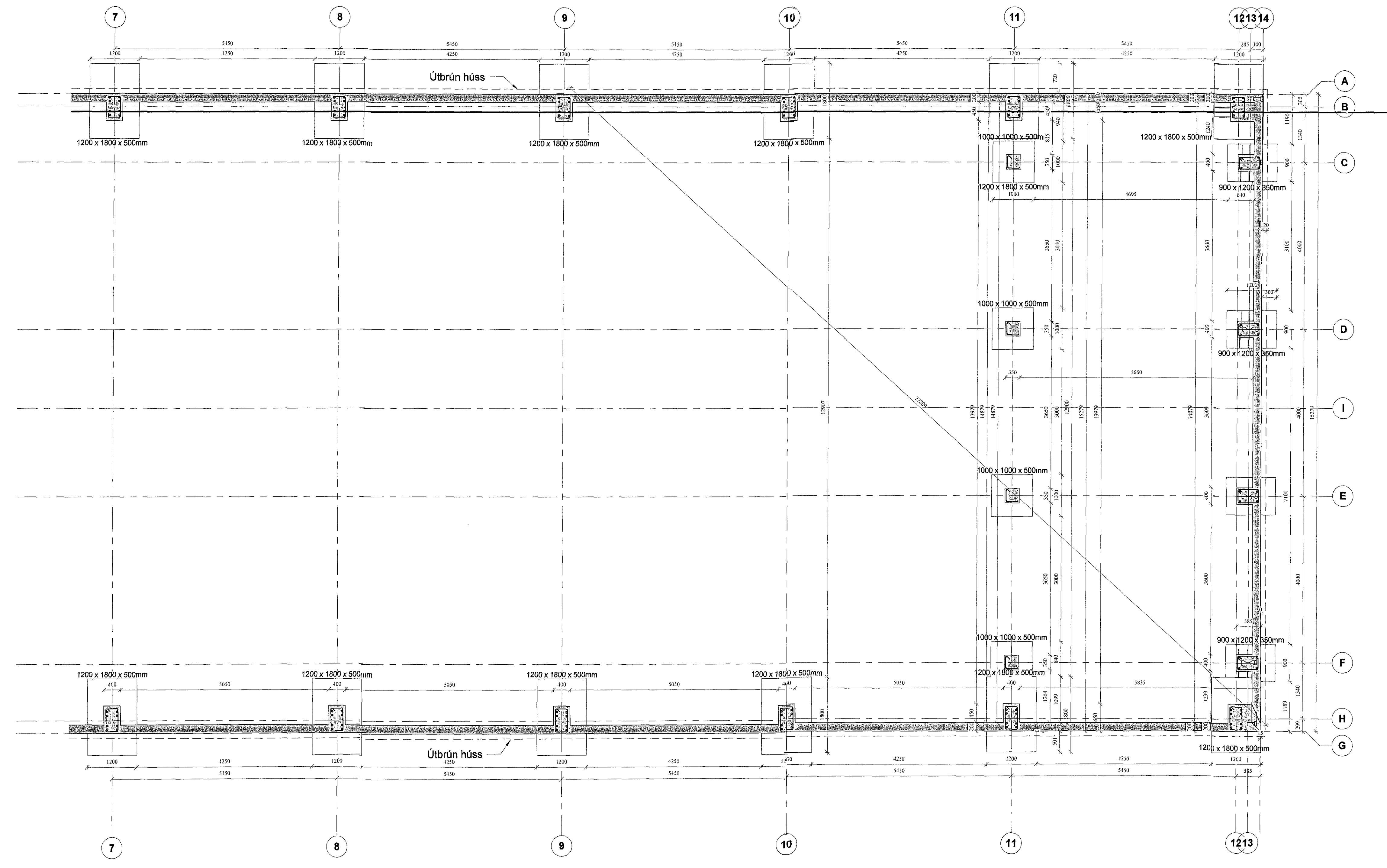
1 SÖKKULLI - NORÐURHLUTI 1 : 50
