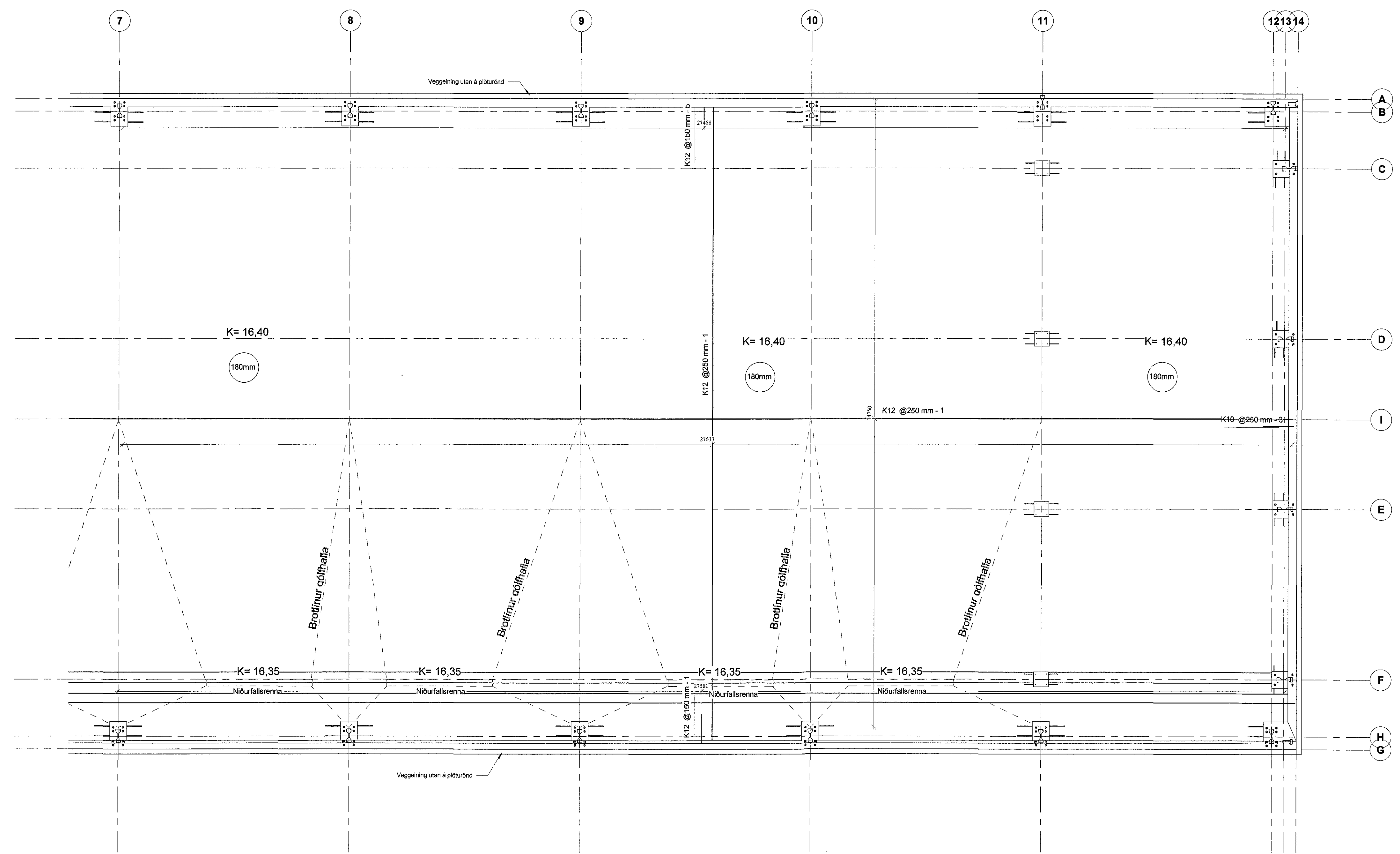
1 BOTNPLATA - NORÐURHLUTI 1:50
