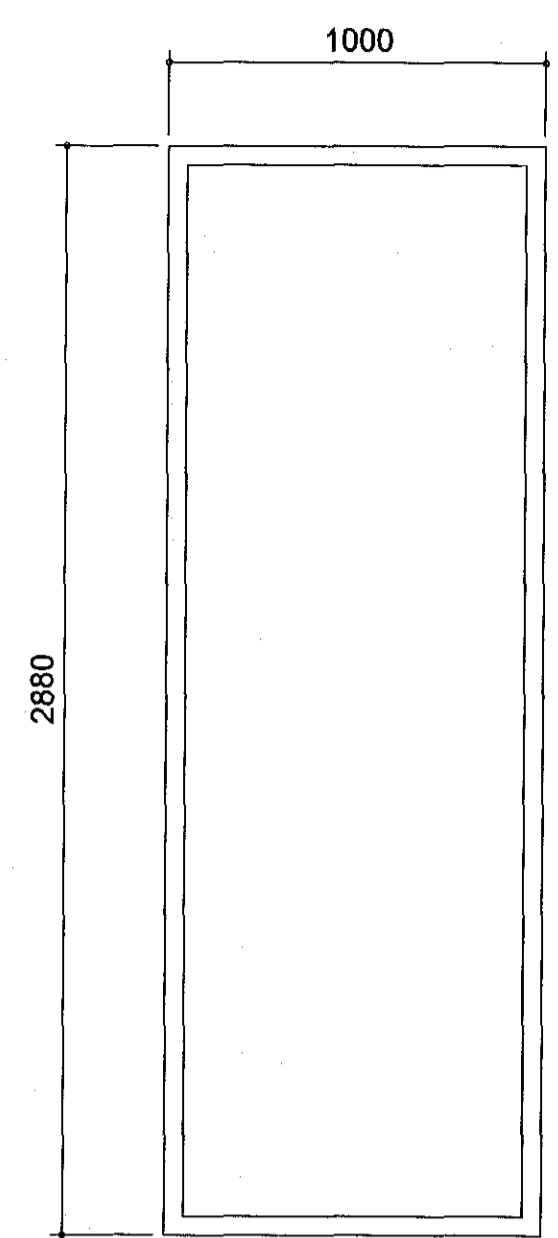
Gluggi nr 3 (eldra hús) 3 stk Litur: RAL 9010
