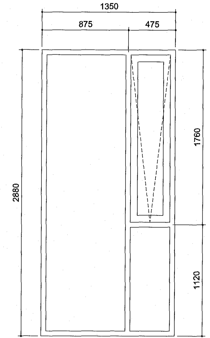
Gluggi nr 1 3 stk Litur: RAL 9010
