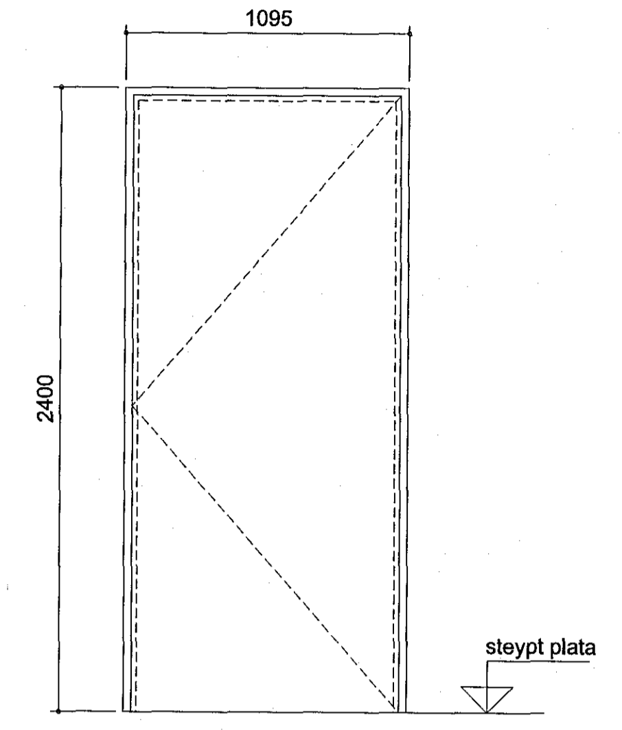
Hurð nr 1 1 stk Litur: RAL 9010
