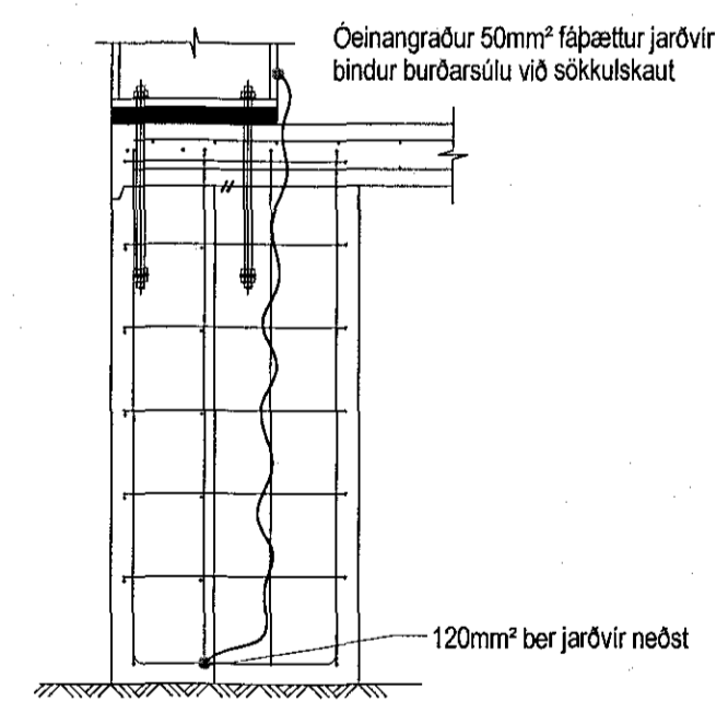
Snið í sökkulskaut 1:20
