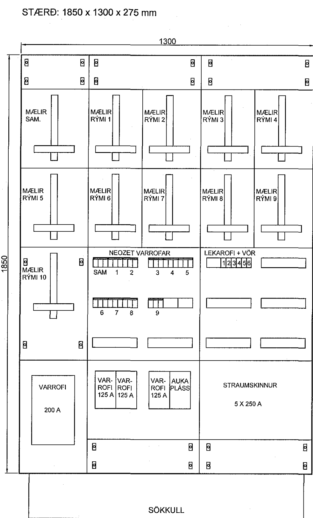
ÚTLIT TÖFLU TA mkv 1:10
