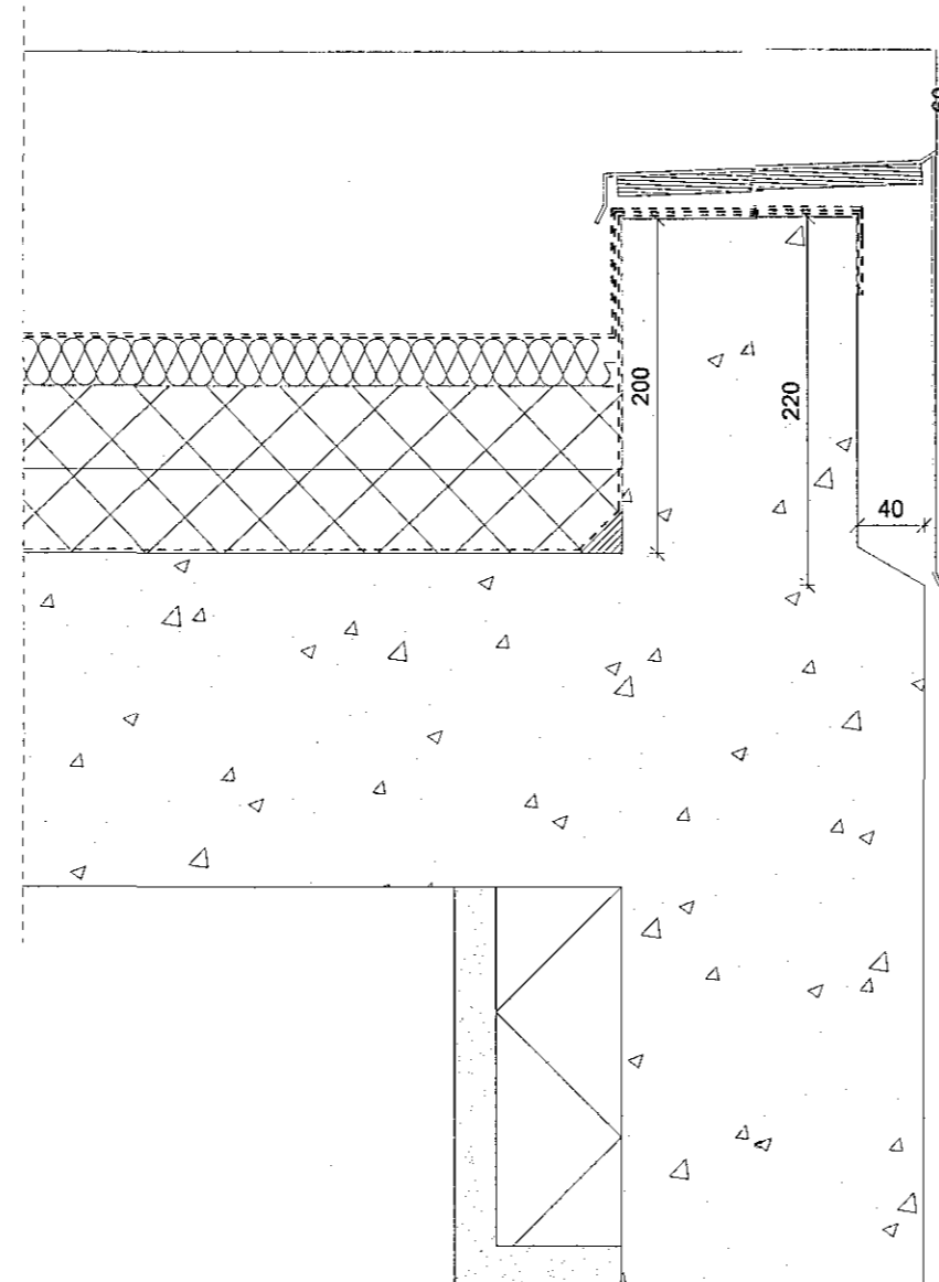
Innfelling í útvegg Lóðrétt hlutasneiðing 1:5
