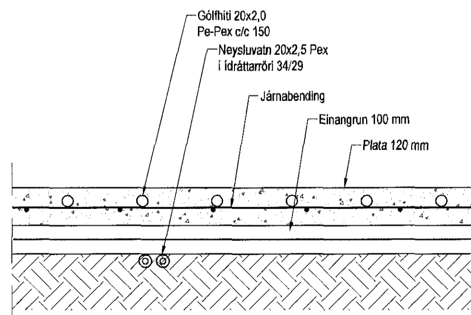
Hita- og vatnslagnir, Snið í botnplötu bílageymslu, 1:10
