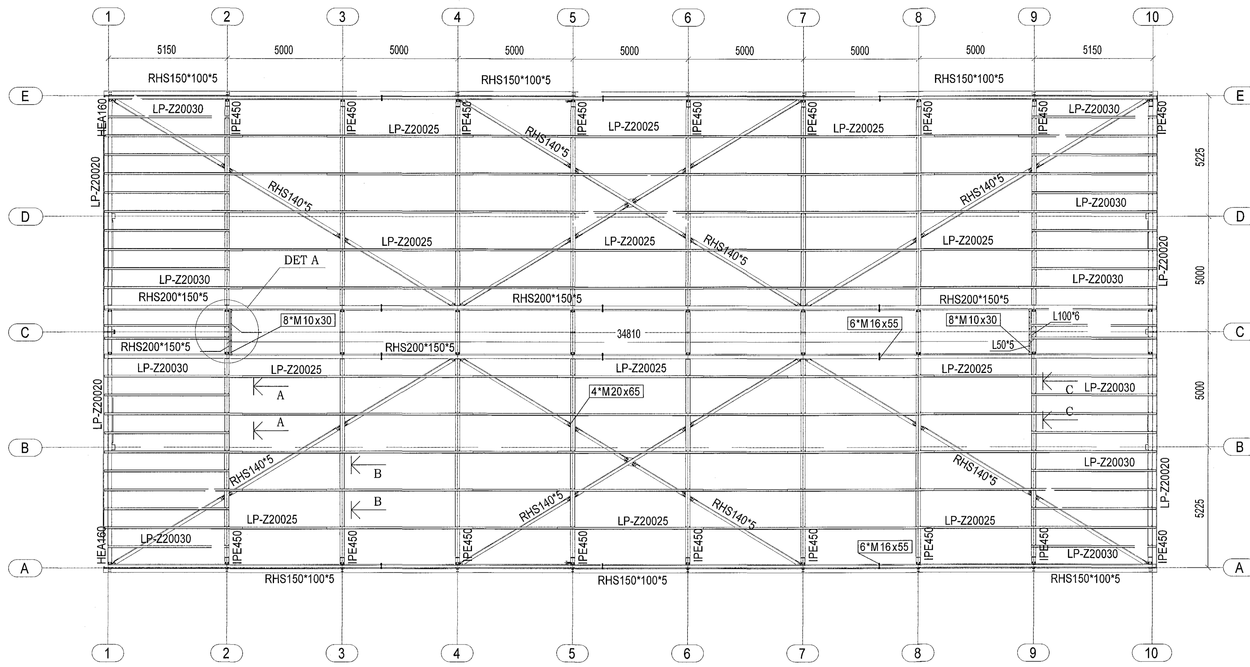
ÞAKMYND 1:100
