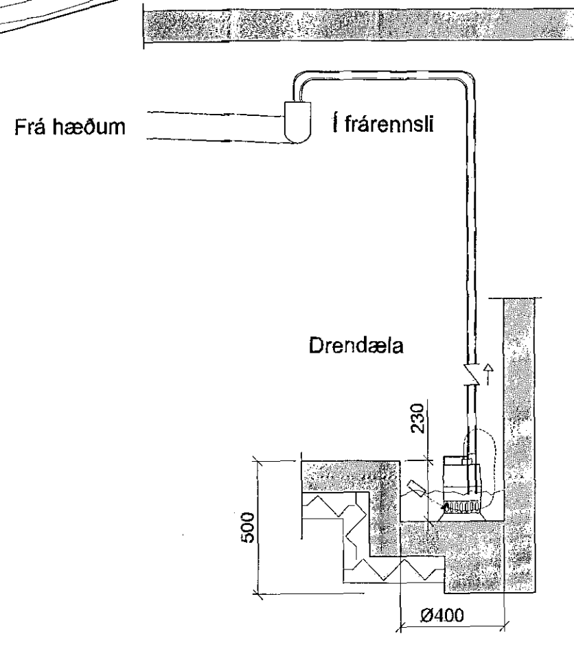
Drendæla (A-A) 1:20
