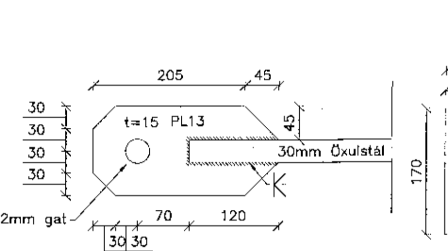
51 Tenging IPE140 bita við reykflúga B(25)01 B(27)01 Mkv: 1:5
