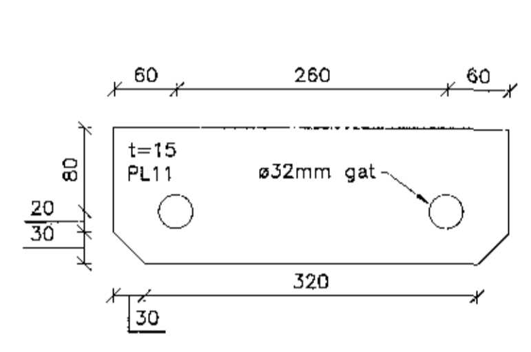
50 Tenging IPE langbita við stálgrind B(25)01 B(27)01 Mkv: 1:5
