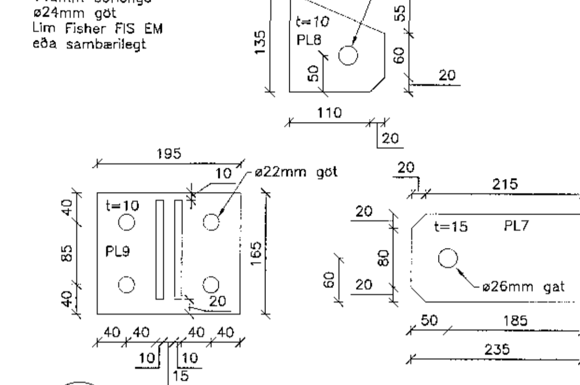
54 Tenging hallandi kassaprófilis við úttegg B(25)01 B(27)01 Mkv: 1:5
