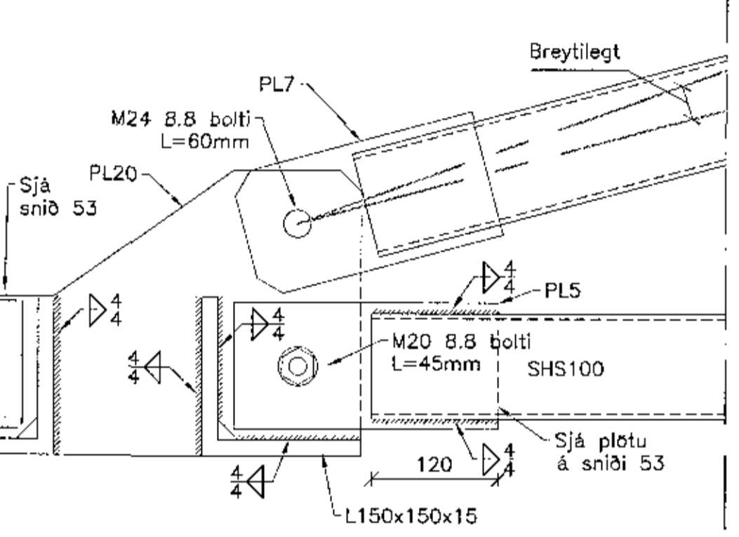
54 Tenging hallandi kassaprófilis við úttegg B(25)01 B(27)01 Mkv: 1:5
