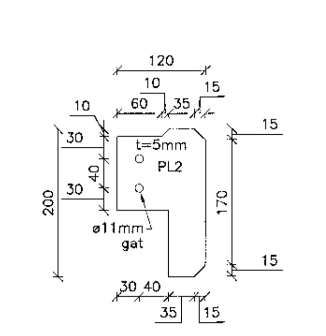
51 Tenging IPE140 bita við reykflúga B(25)01 B(27)01 Mkv: 1:5
