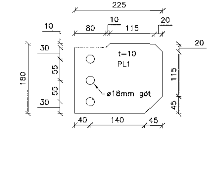
50 Tenging IPE langbita við stálgrind B(25)01 B(27)01 Mkv: 1:5
