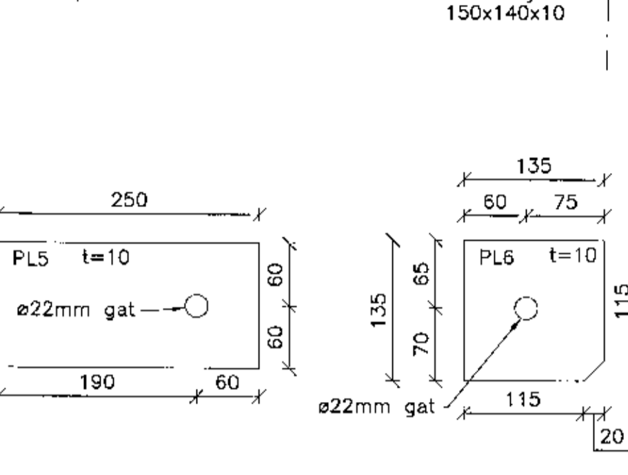
53 Tenging kassaprófilis við stálgrind B(25)01 B(27)01 Mkv: 1:5
