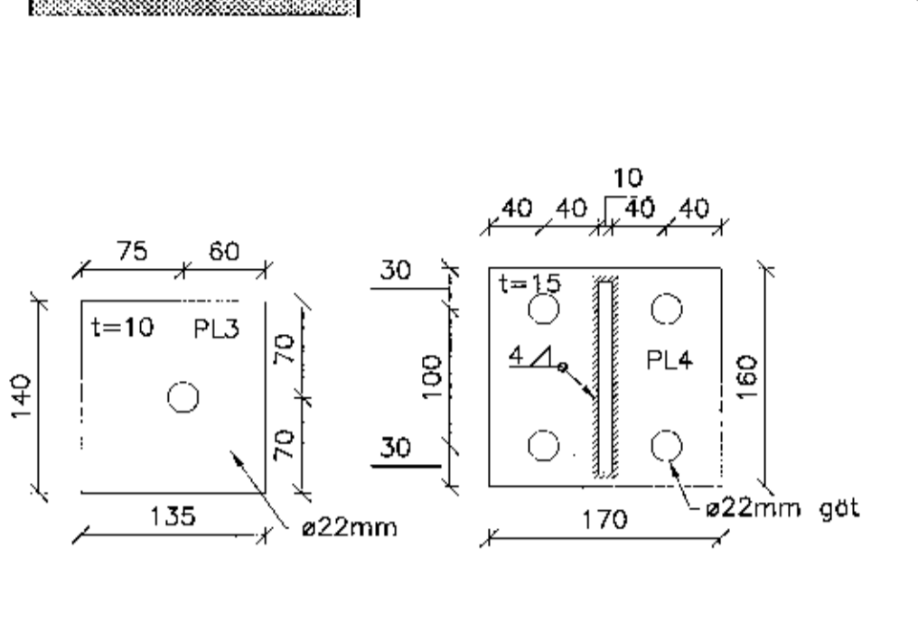
52 Tenging kassaprófilis við úttegg B(25)01 B(27)01 Mkv: 1:5
