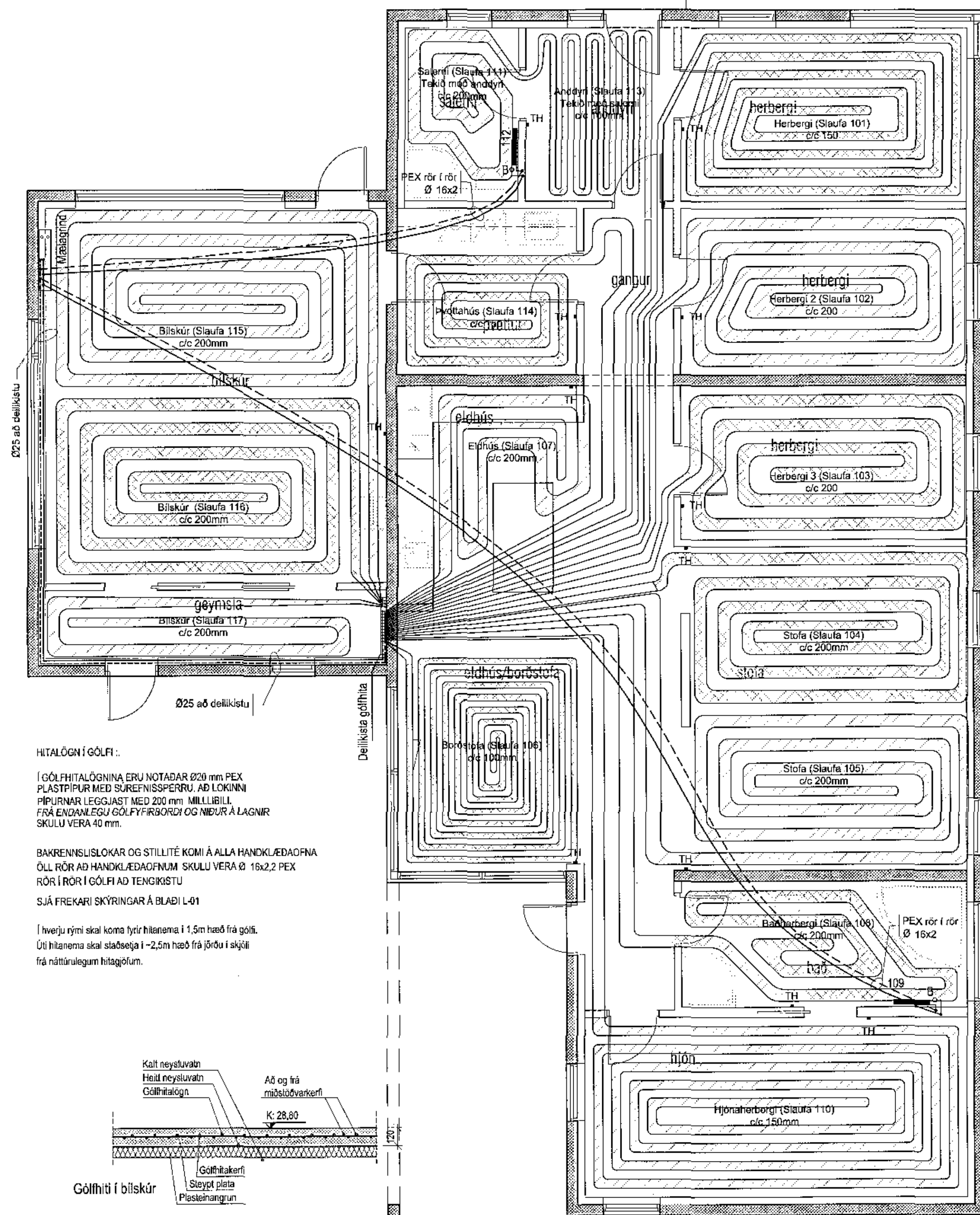
Grunnmynd miðstöðvarlagna 1:50
