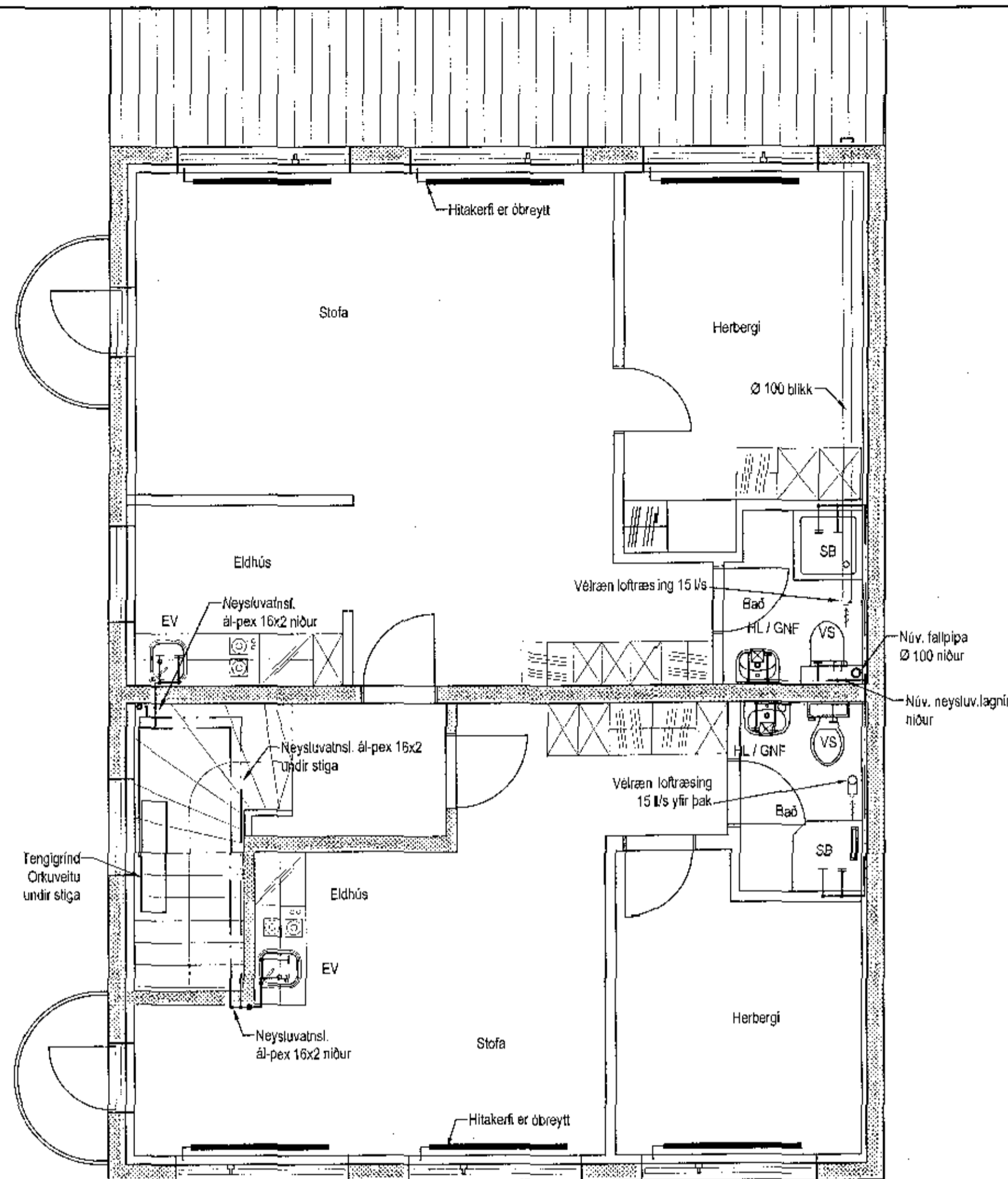
Neyslu- og fráveitulagnir 2. hæð, 1:50
