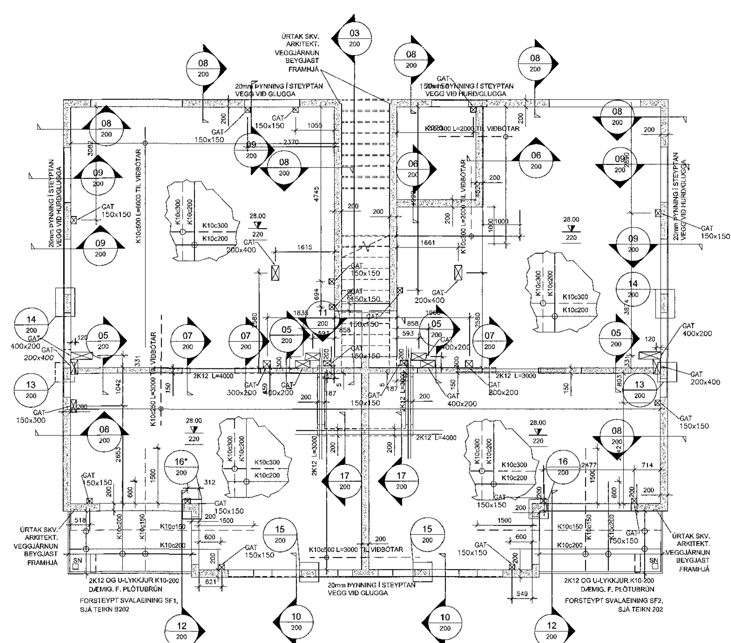
VEGGIR OG LOFTAPLATA 1.HÆÐAR, GRUNNMYND MKV. 3
