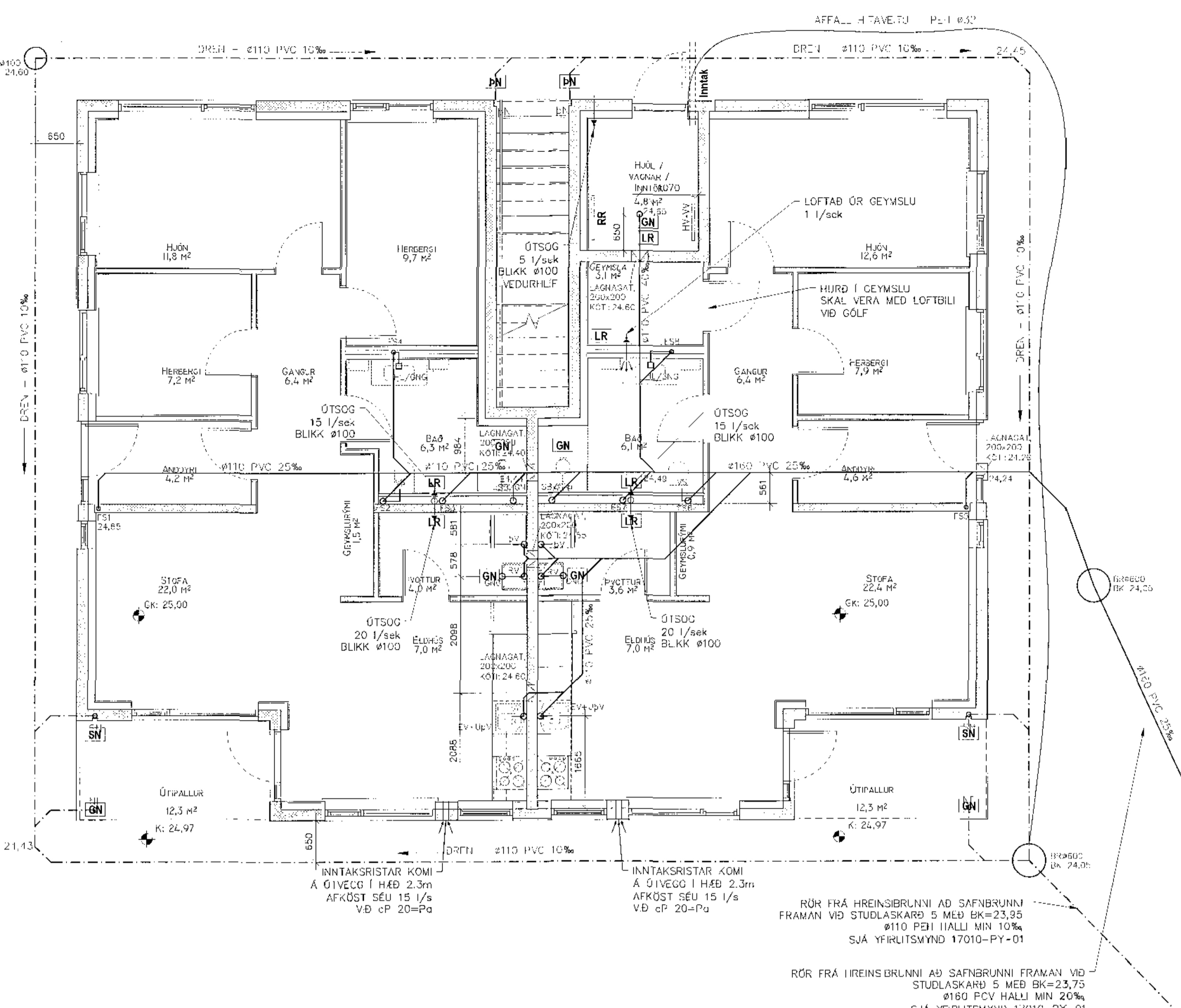
GRUNNMYND 1.HÆÐ MKV.3
