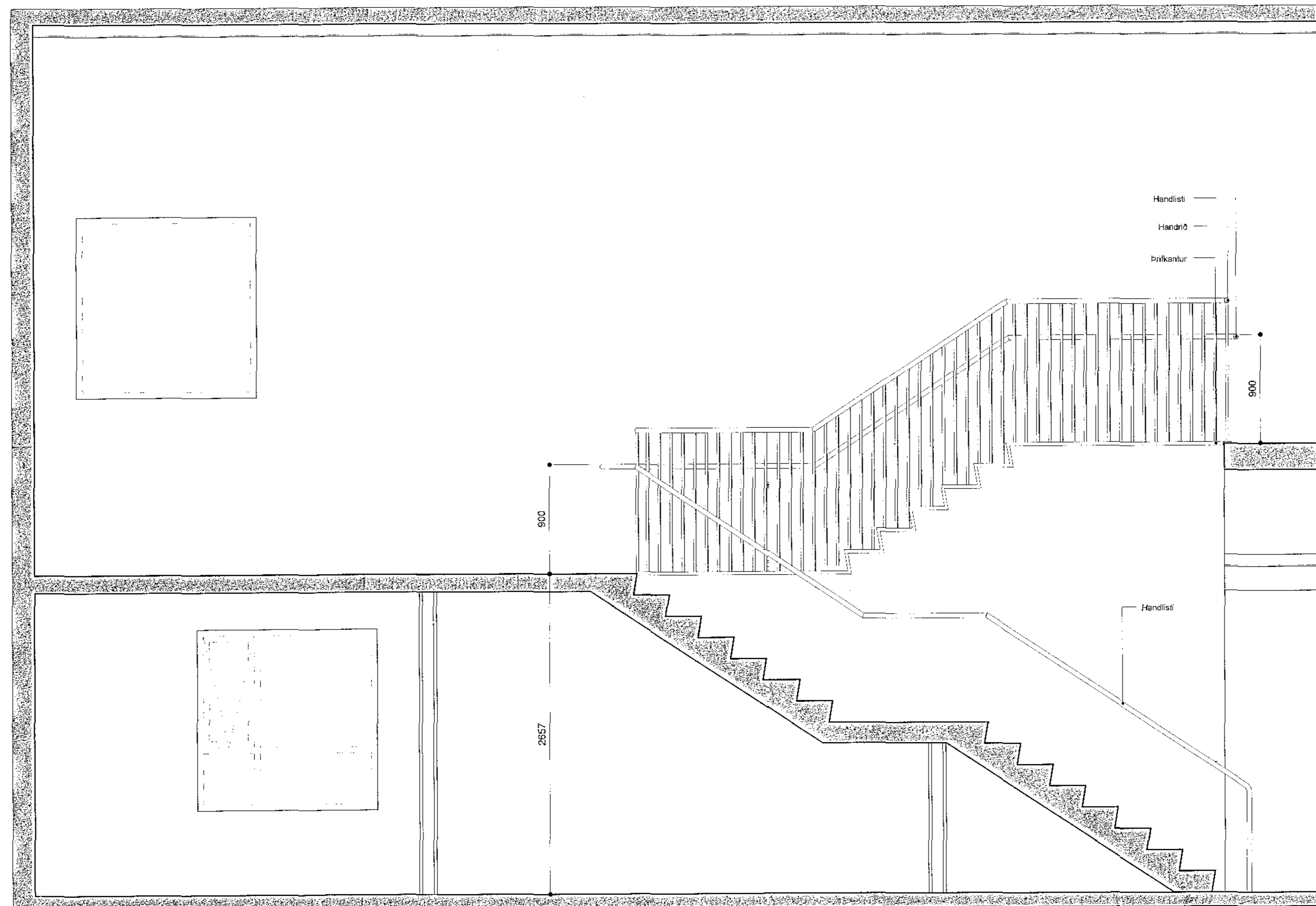
Snið 2 mkv: 1 : 20
