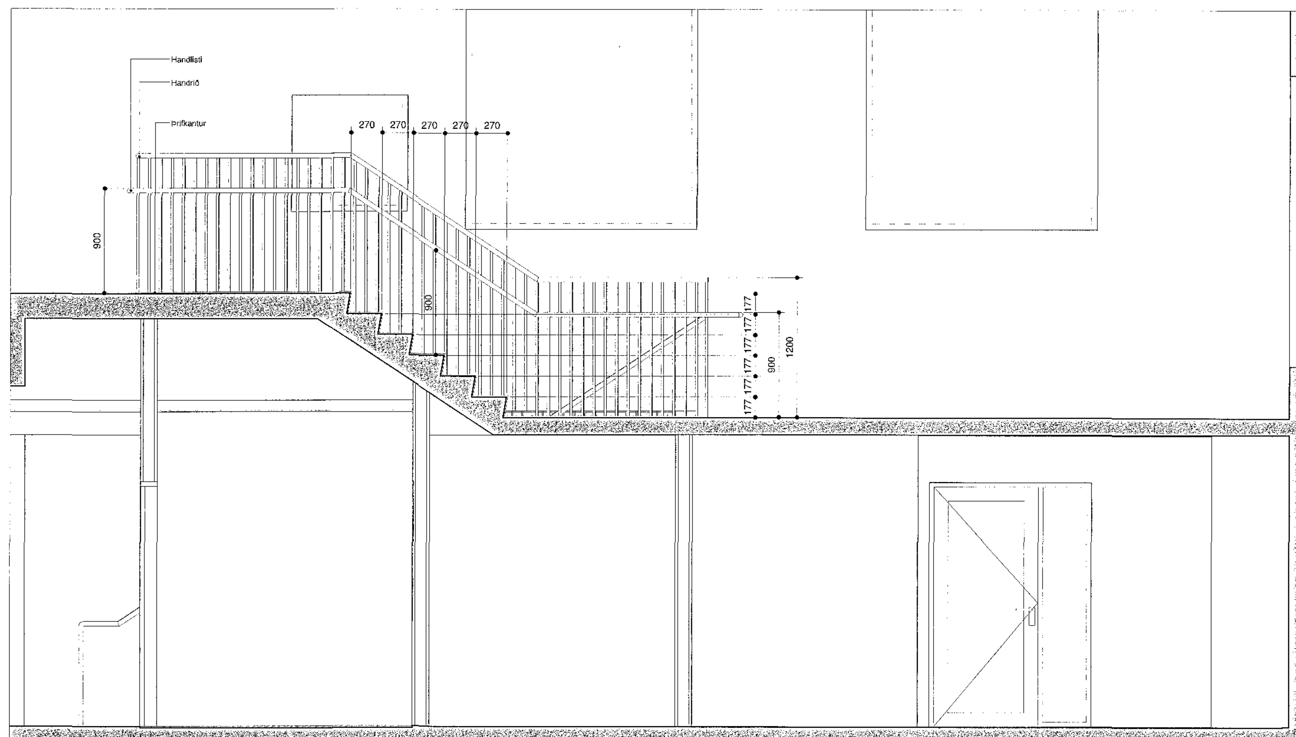
Snið 4 mkv: 1 : 20
