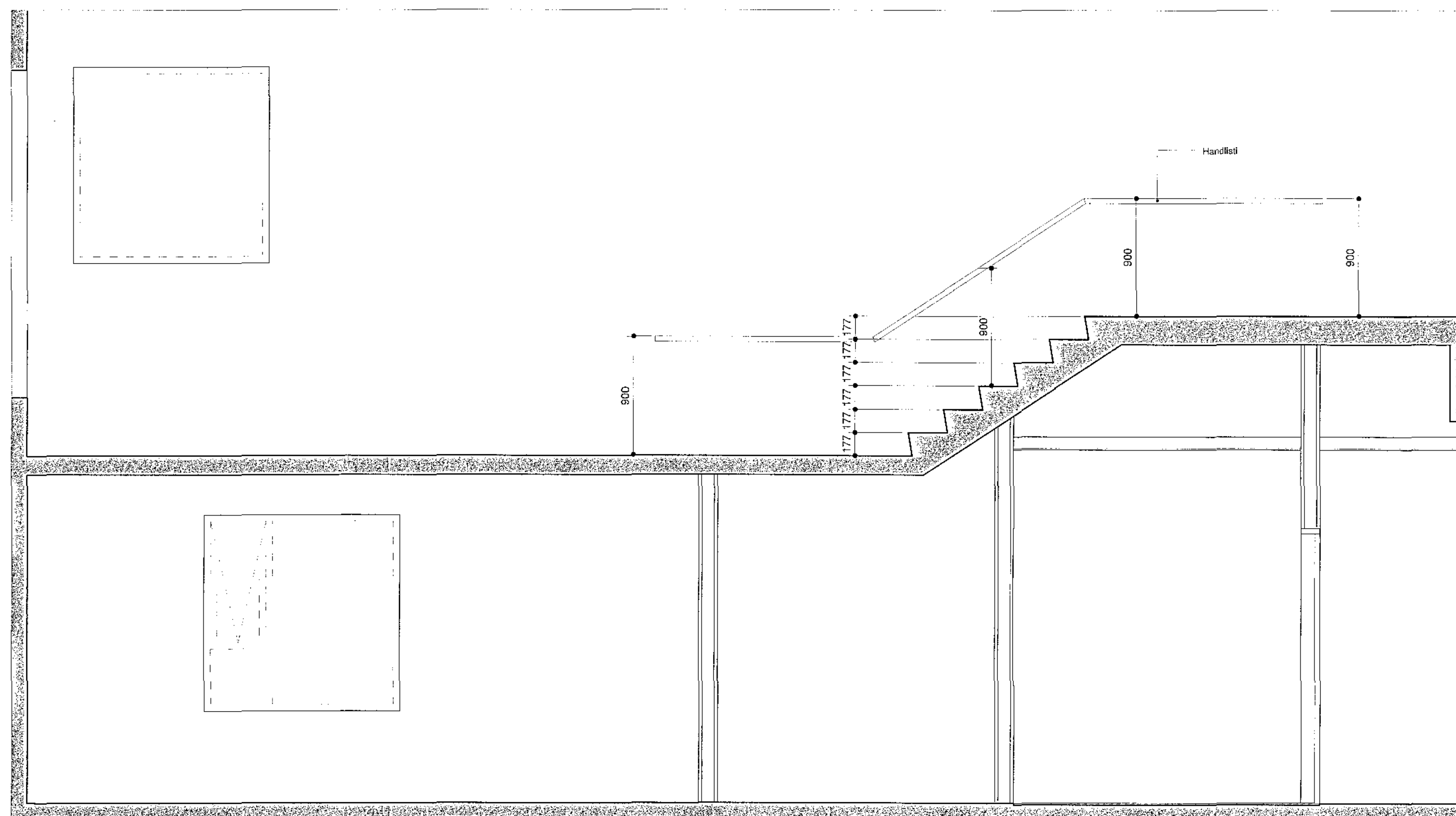
Snið 5 mkv: 1 : 20
