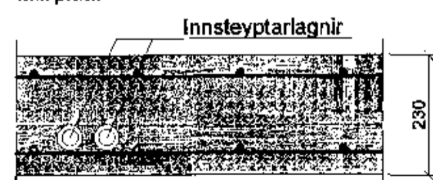
Innsteyptar lagnir 1:10 Milliplata
