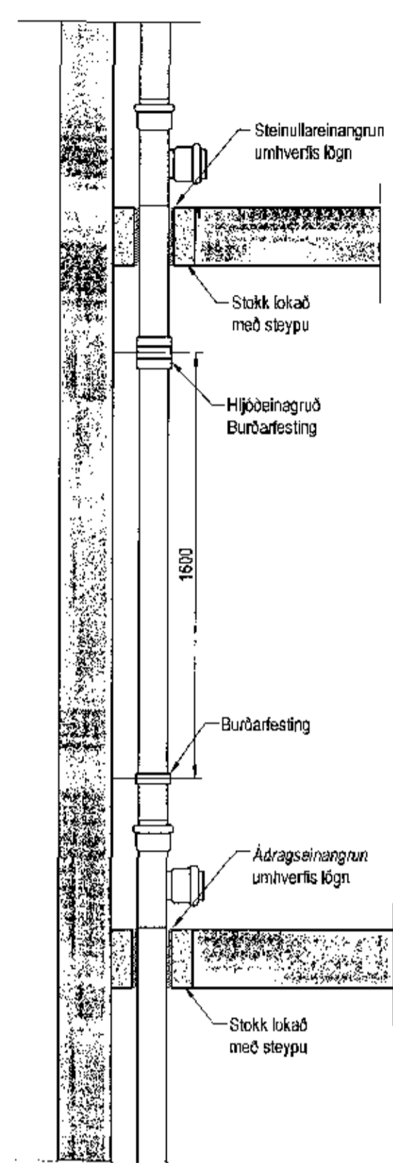
Fallþípa, festingar 1:20
