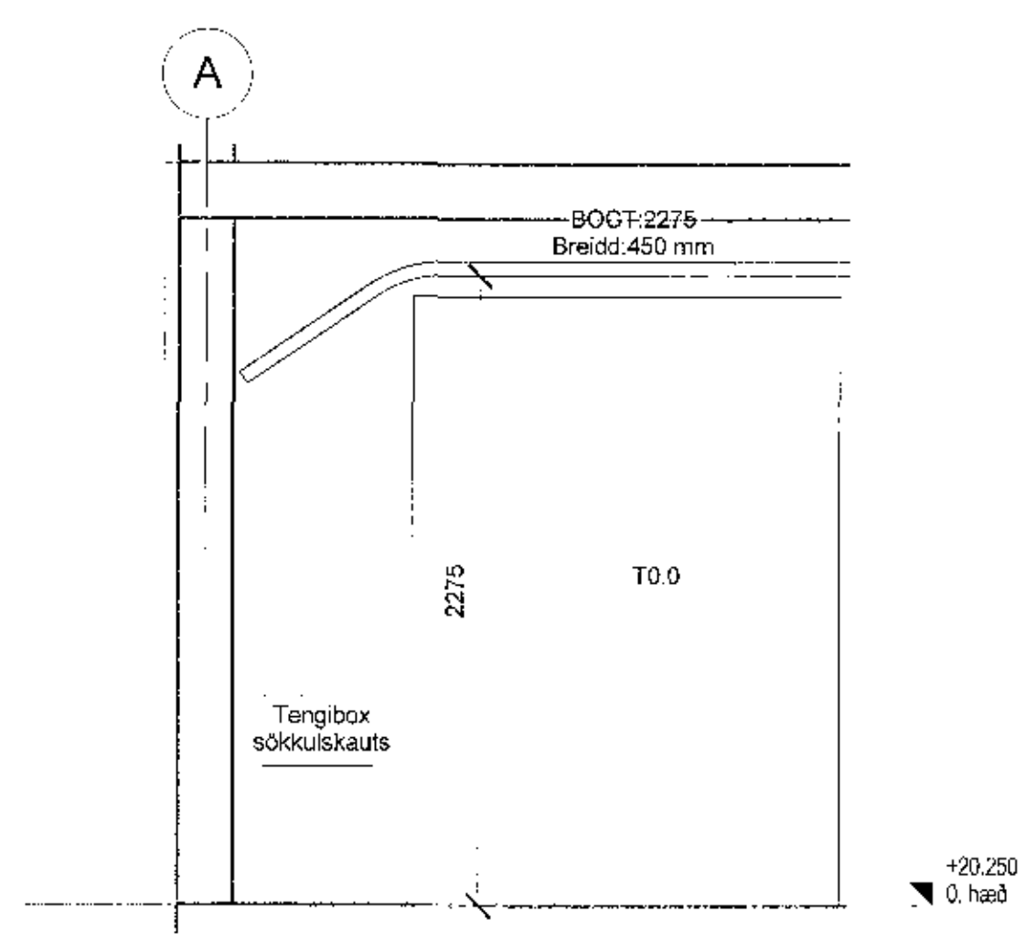
A-A Snið_14 A-A 0,3,4,0 1:25
