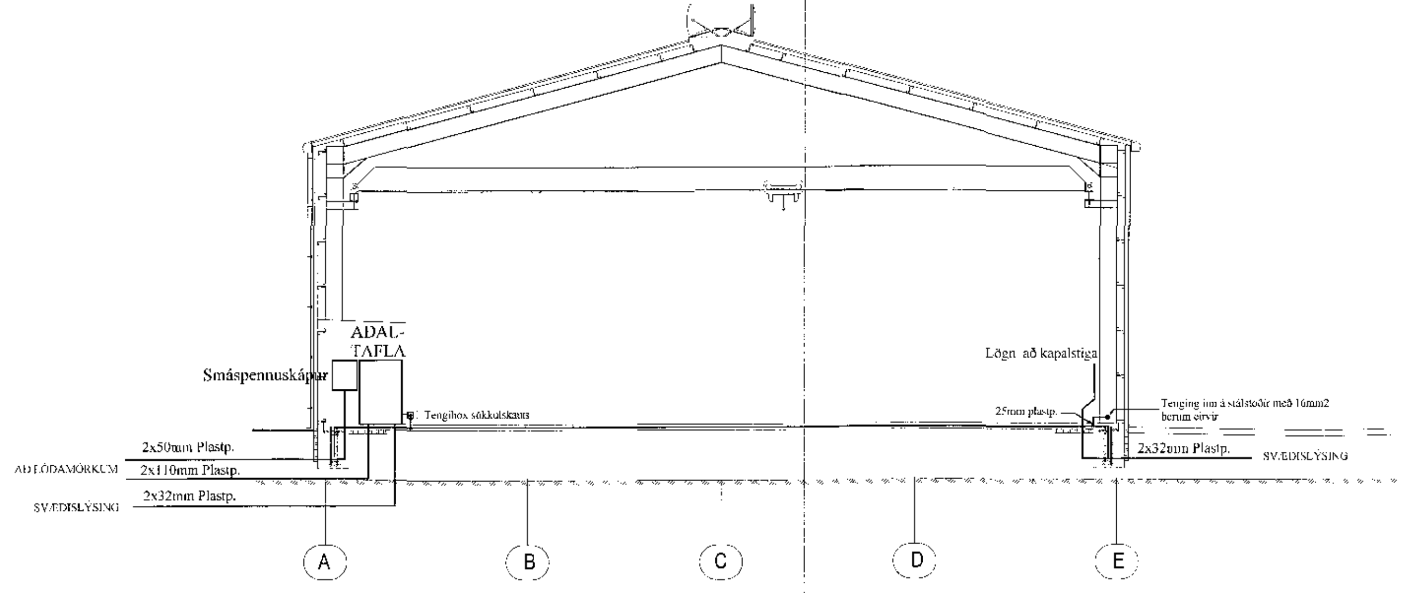
SNIÐ A-A Í INNTAK M 1:100
