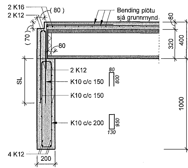
B39 Snið 1 : 20
