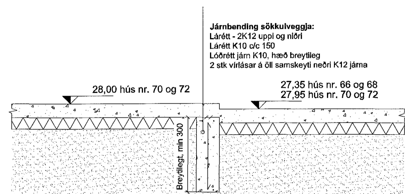
03 Snið, innveggir sökkla við bílskúr 101B 1:20
