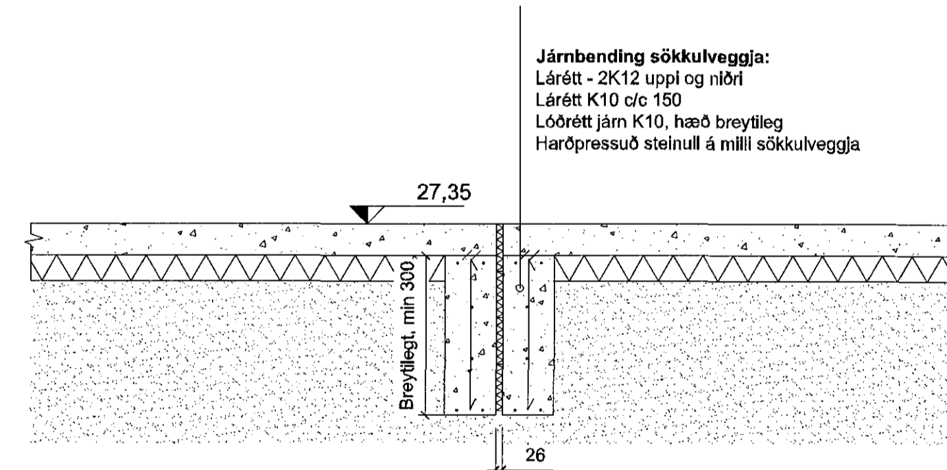
04 Snið, sökkjar milli húsa nr. 66 og 68 101B 1:20
