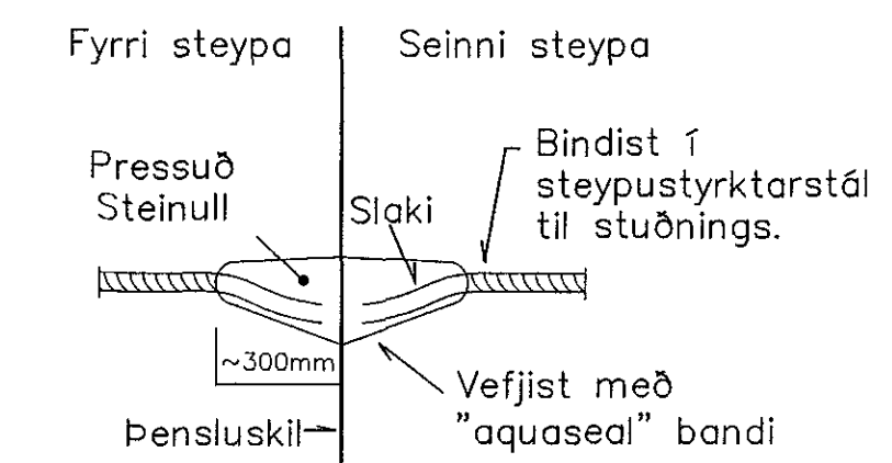
SÉRMYND G VERNDUN JARÐTAUGA Á ÞENSLUSKILUM ÞAR SEM VIÐ Á
