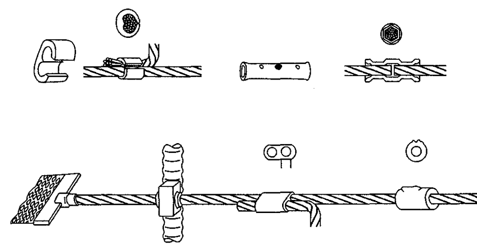
SÉRMYND A DÆMIGERÐAR TENINGAR JARÐTAUGA ÓHEIMILT ER AÐ NOTA VÍRALÁSA TIL TENINGA JARÐTAUGA OG STEYPUTEINA
