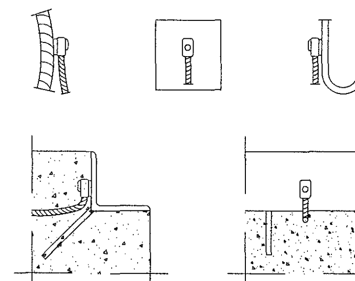
SÉRMYND F SÖÐIN TENING JARÐTAUGA Í STÁLRAMMA.
