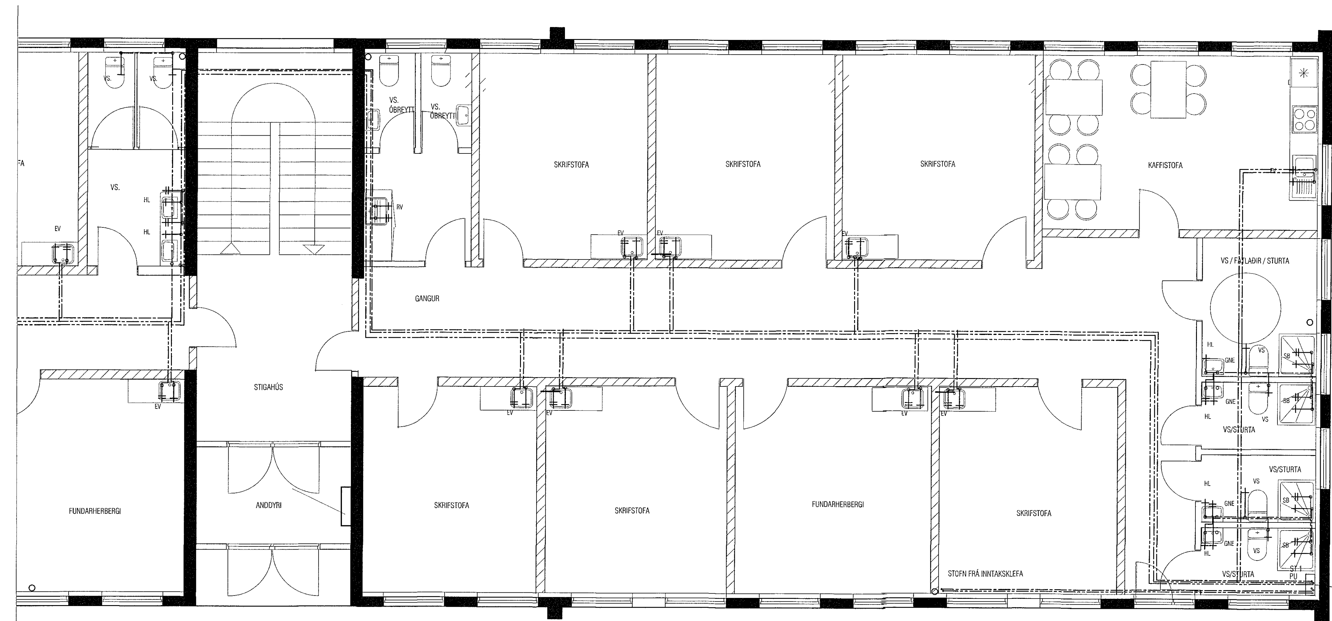
GRUNNMYND 2. HÆÐAR TIL HÆGRI, NEYSLUVATN MKV. 1:50
