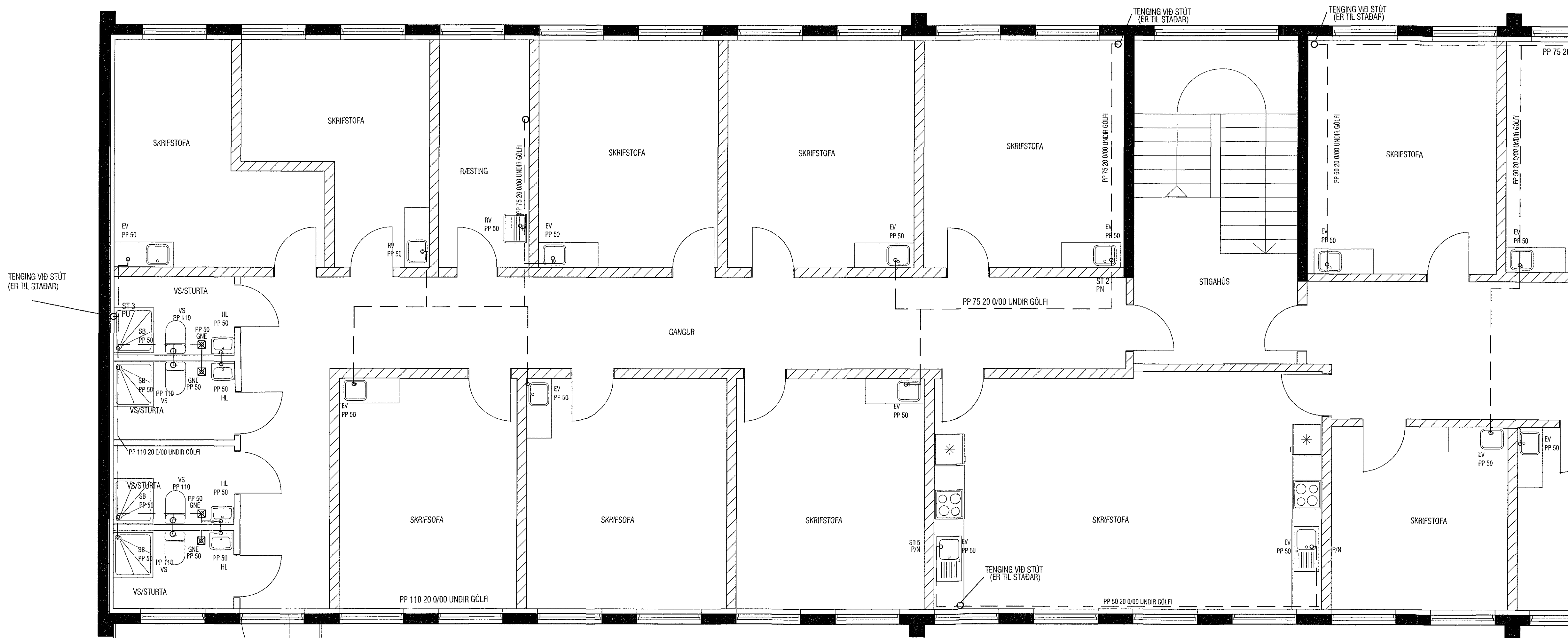
GRUNNMYND 3. HÆÐAR TIL VINSTRI, FRÁRENNSLI MKV. 1:50
