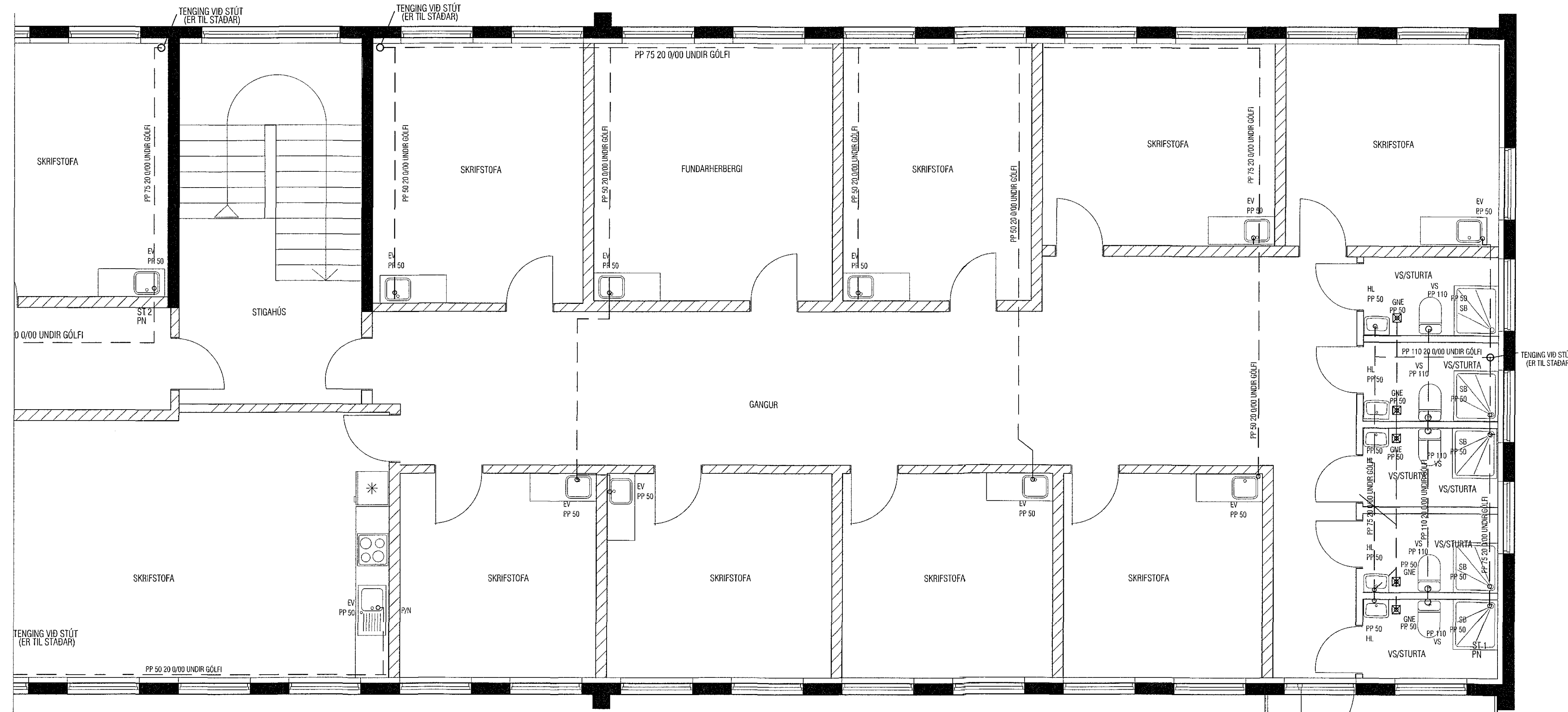
GRUNNMYND 3. HÆÐAR TIL HÆGRI, FRÁRENNSLI MKV. 1:50
