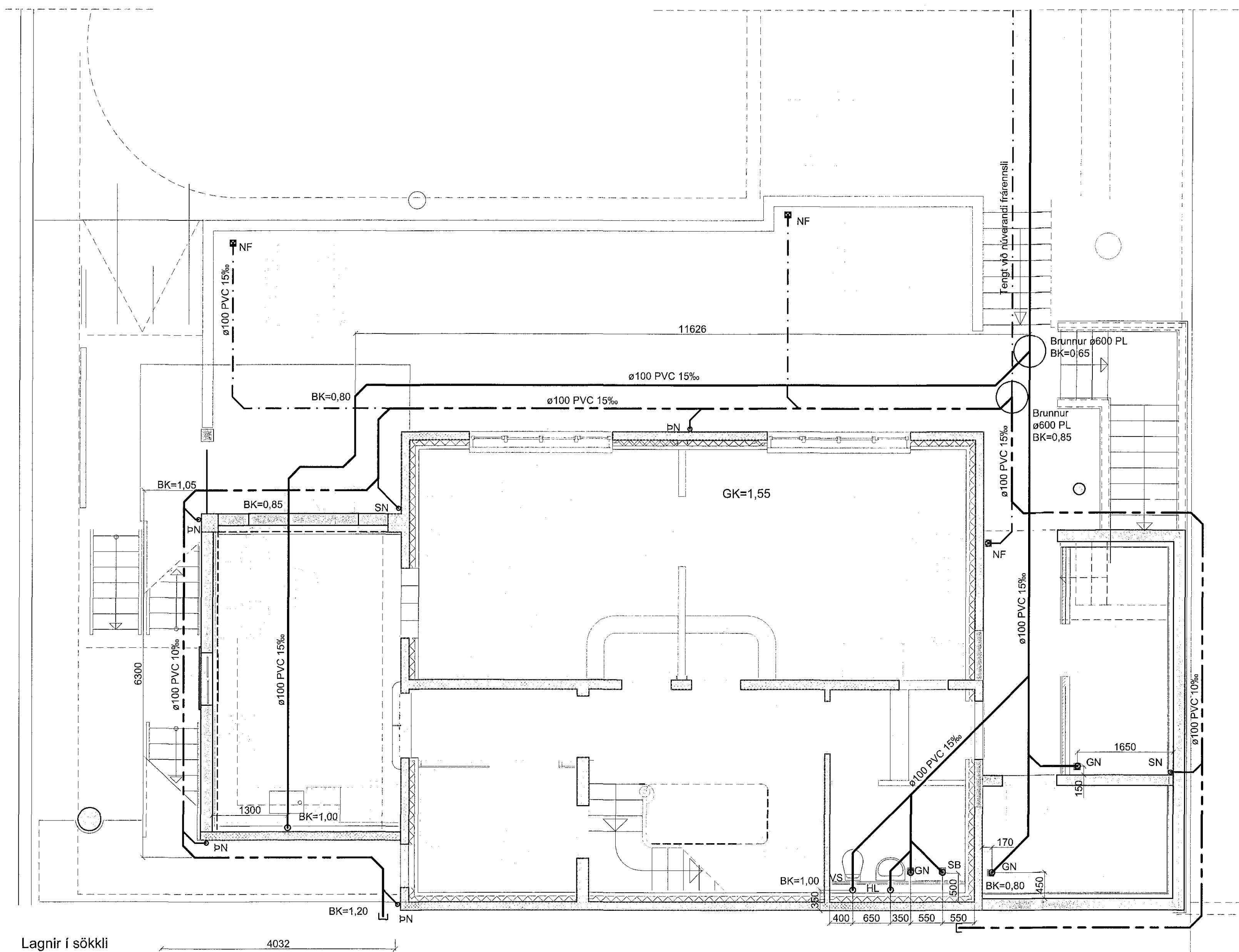
Lagnir í sökkli Mkv. 1:50
