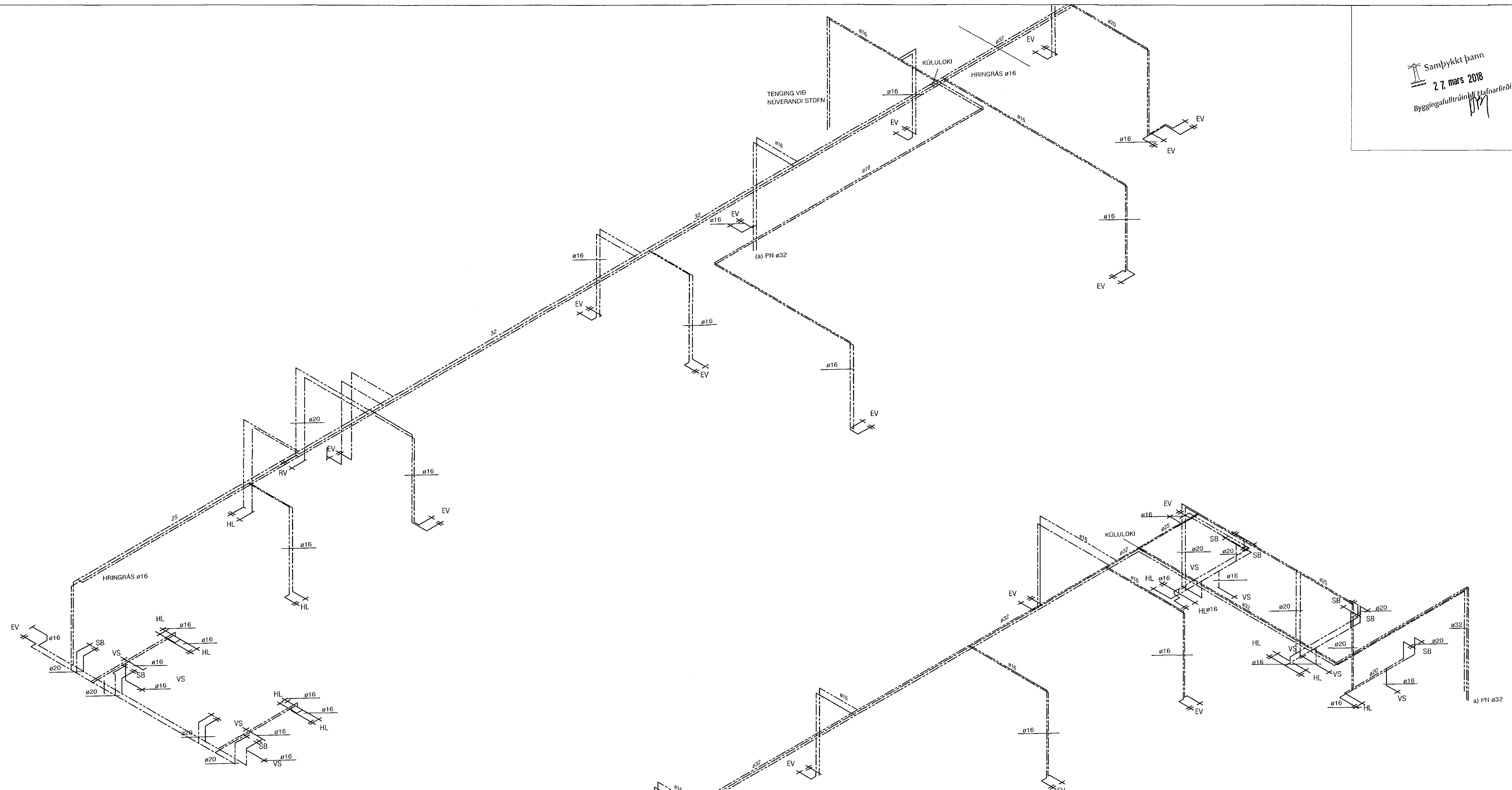
RÚMMYND 3. HÆÐAR TIL VINSTRI NEYSLUVATN MKV. 1:50
