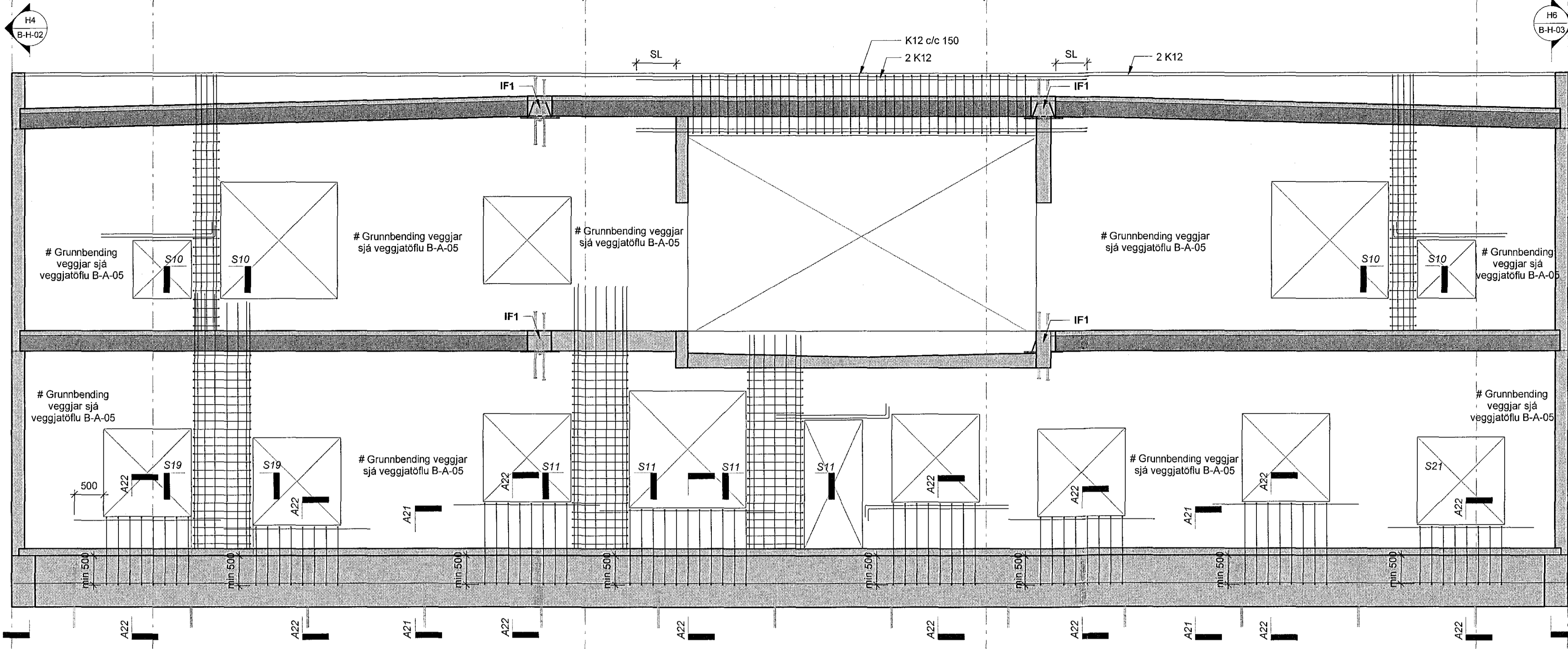
H5 V-A-02 1 : 50
