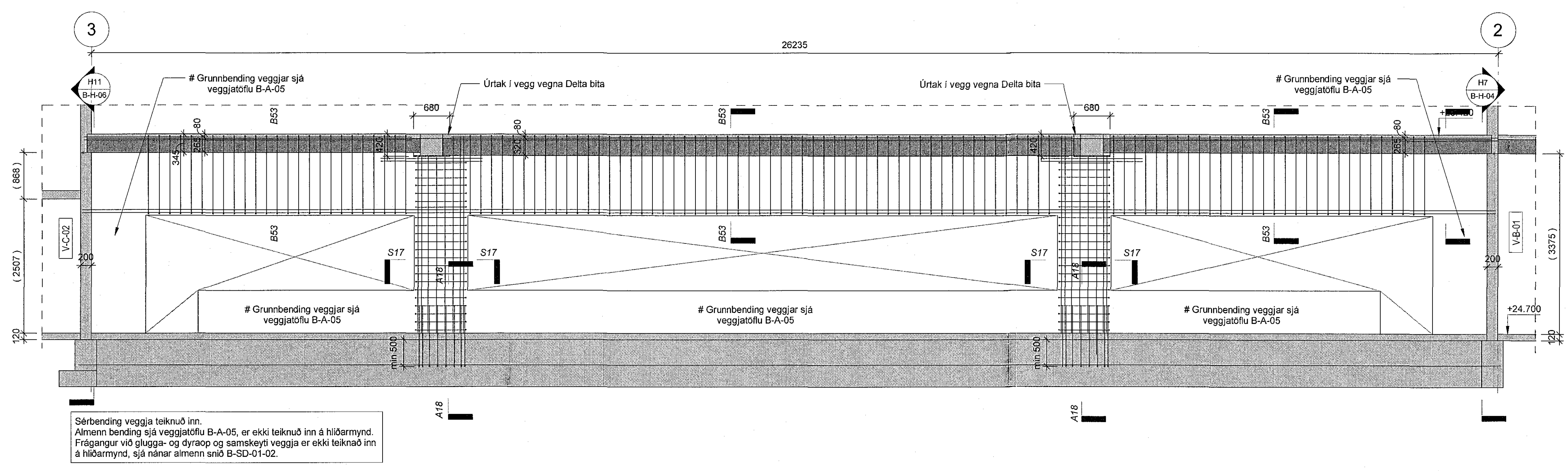
H9 V-B-01 1 : 50
