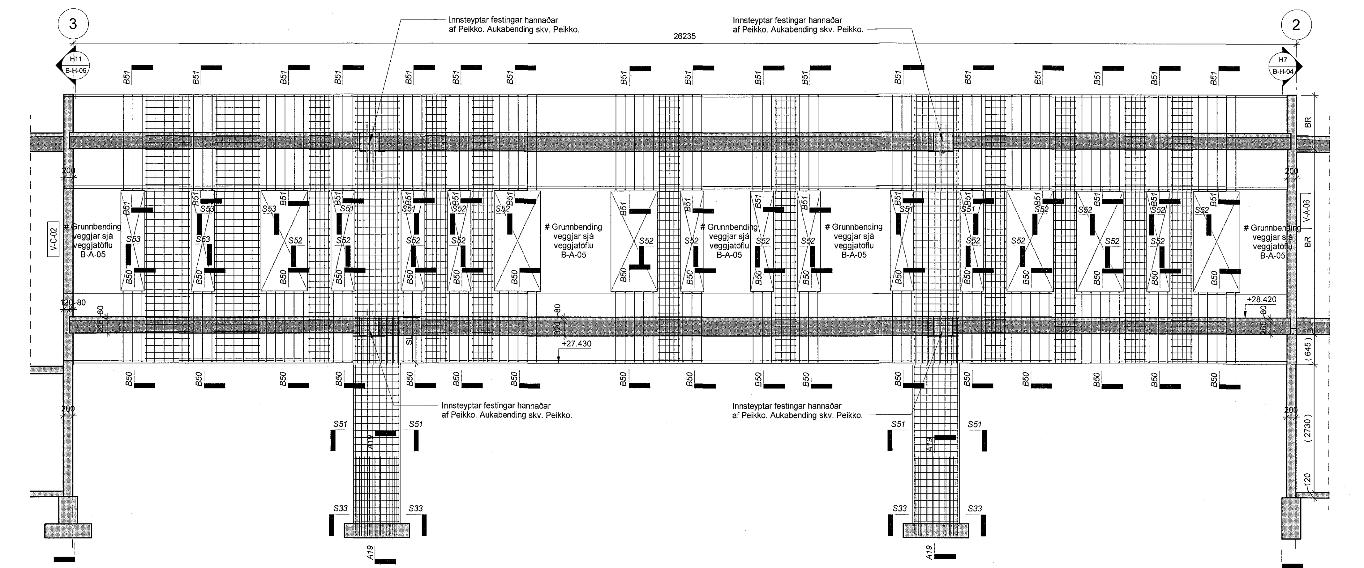
H10 V-B-06 1 : 50
